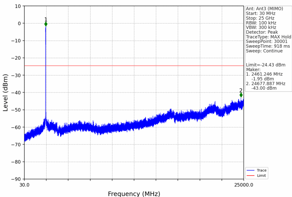
802.11n(HT40)_HCH_2452MHz_Ant3 (MIMO)_NTNV
