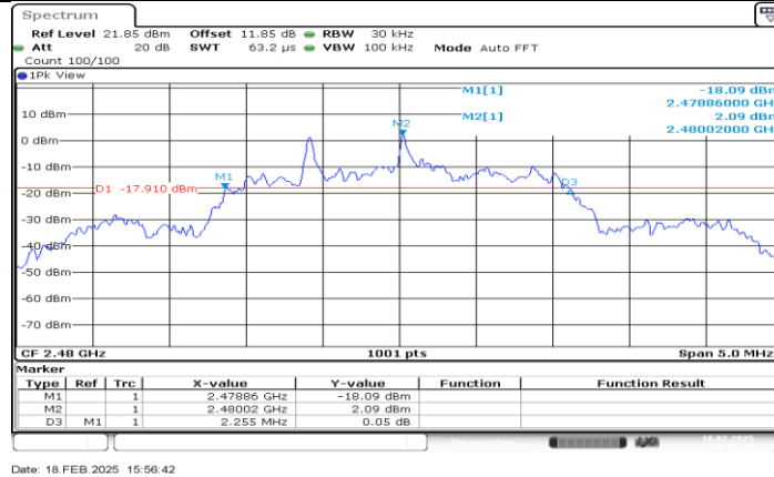
SRD 2.4G_Ant1_2480
