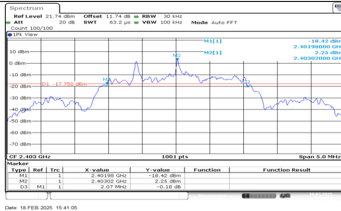
SRD 2.4G_Ant1_2403
