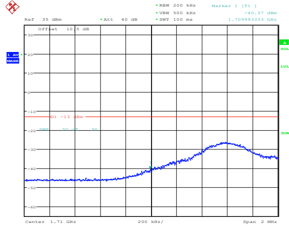
Band4-10MHz-QPSK-20000-50RB#0
