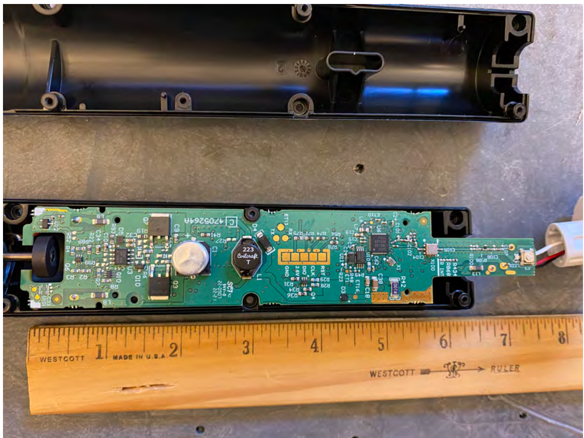
Top PCB
