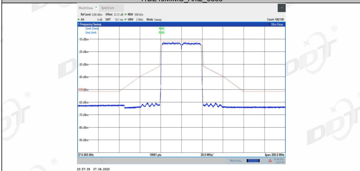
11BE40MIMO_Ant3_6565
