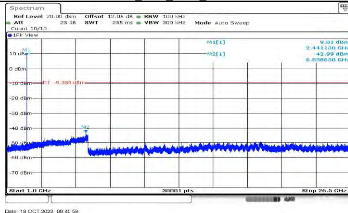
3DH5_Ant0_2441_1000~26500
