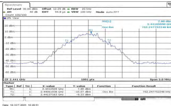
DH5_Ant1_2441
