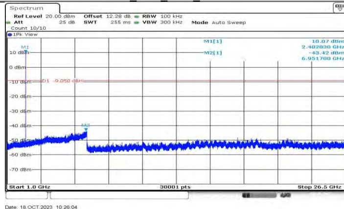
DH5 Ant1 2402 1000~26500
