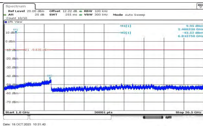
DH5 Ant1 2480 1000~26500
