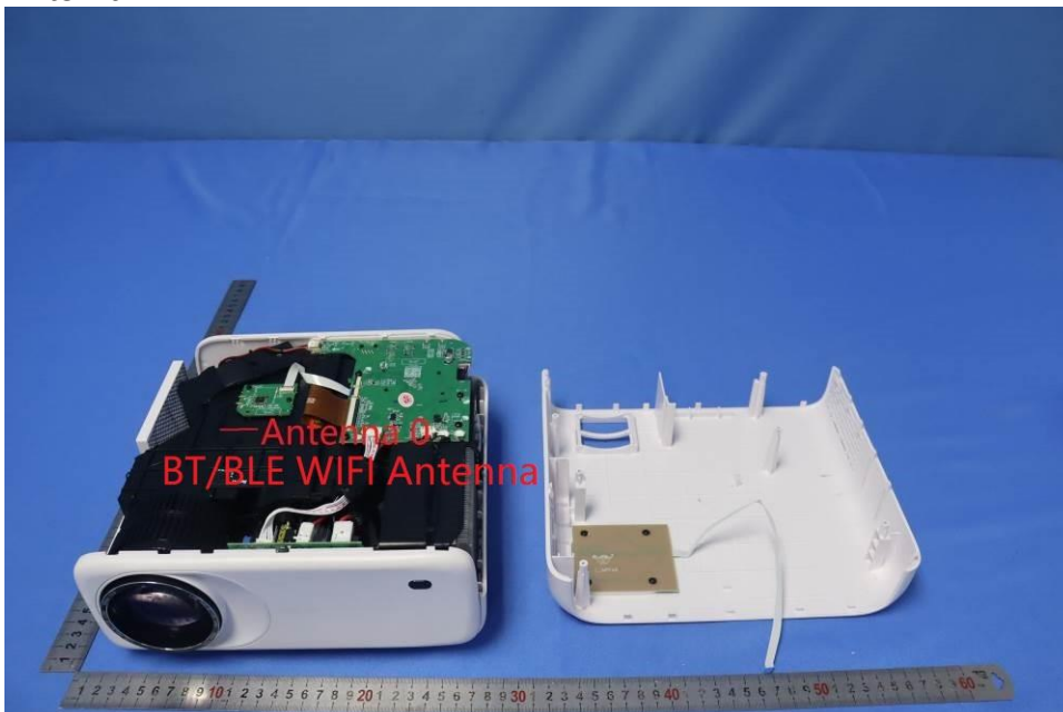
Antenna
