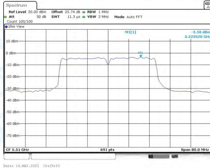
11AC40MIMO_Ant3_5510
