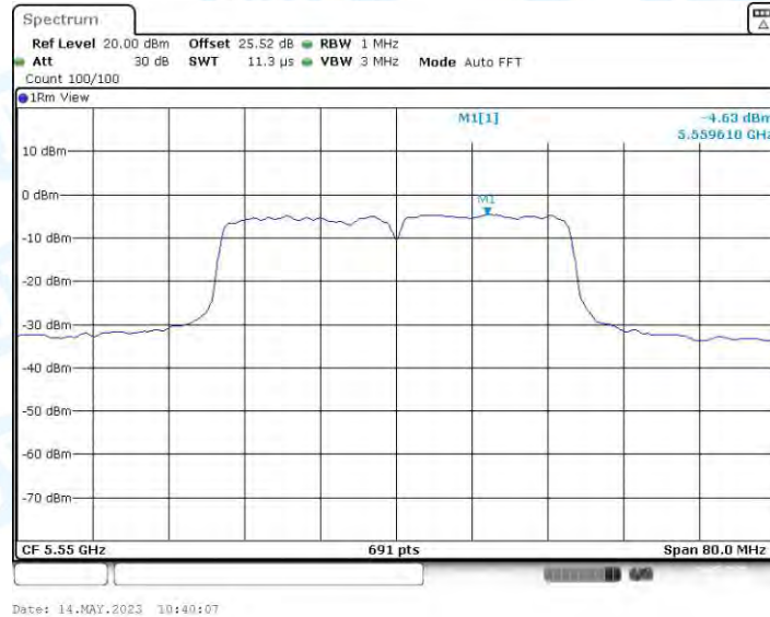
11N40MIMO_Ant3_5550
