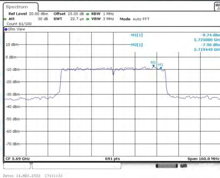
11AC80MIMO_Ant2_5690_UNII-2C
