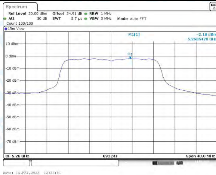
11AC20MIMO_Ant4_5260
