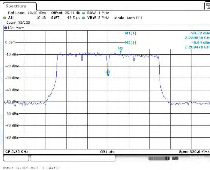
11AC160MIMO_Ant3_5250_UNII-2A
