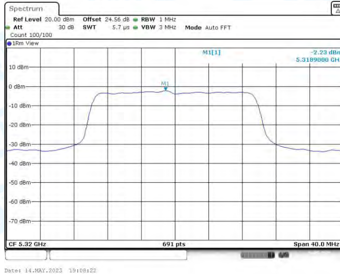
11AX20MIMO_Ant2_5320
