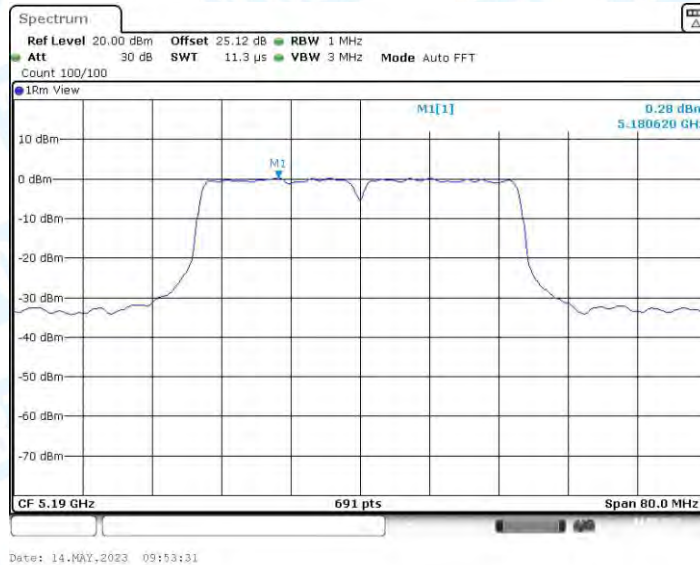
11N40MIMO_Ant3_5190
