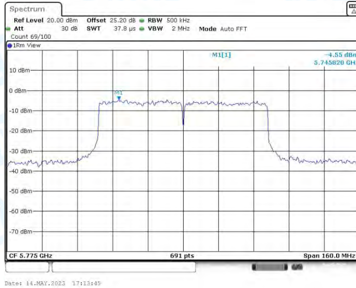
11AC80MIMO_Ant4_5775
