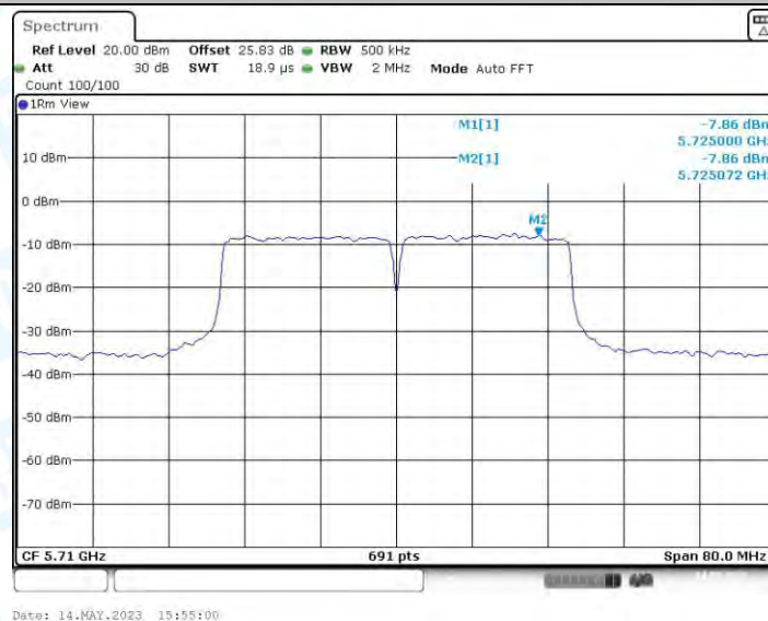
11AC40MIMO_Ant3_5710_UNII-3
