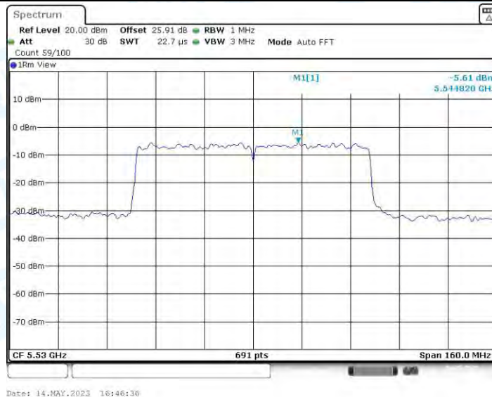
11AC80MIMO_Ant3_5530
