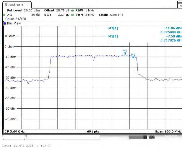
11AC80MIMO_Ant3_5690_UNII-2C
