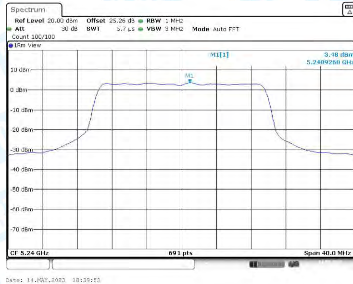
11AX20MIMO_Ant3_5240
