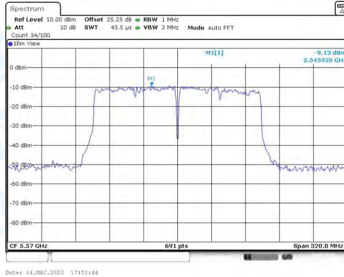
11AC160MIMO_Ant4_5570
