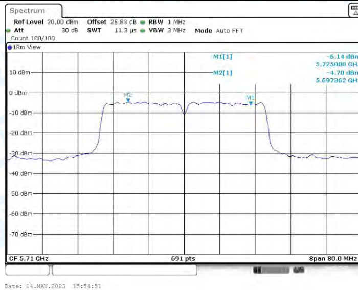
11AC40MIMO_Ant3_5710_UNII-2C
