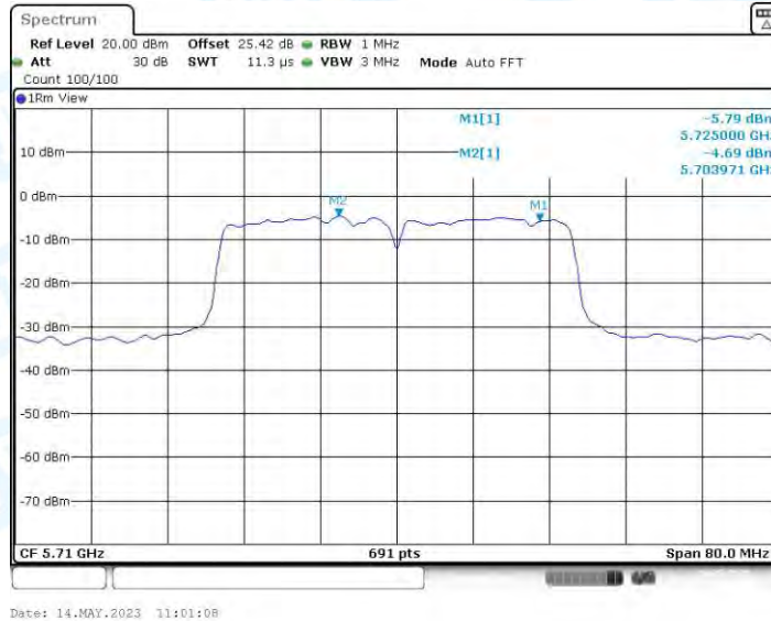
11N40MIMO_Ant4_5710_UNII-2C
