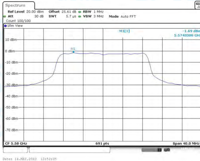
11AC20MIMO_Ant3_5580
