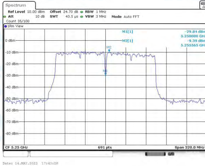
11AC160MIMO_Ant2_5250_UNII-2A
