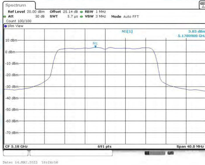
11AX20MIMO_Ant3_5180
