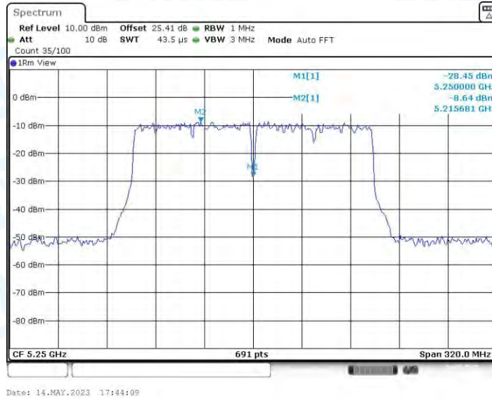
11AC160MIMO_Ant3_5250_UNII-1
