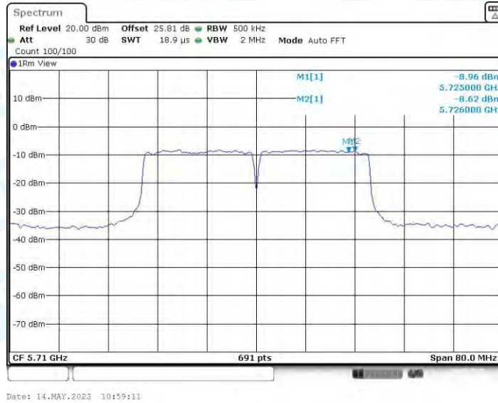
11N40MIMO_Ant3_5710_UNII-3
