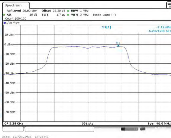
11AC20MIMO_Ant3_5280
