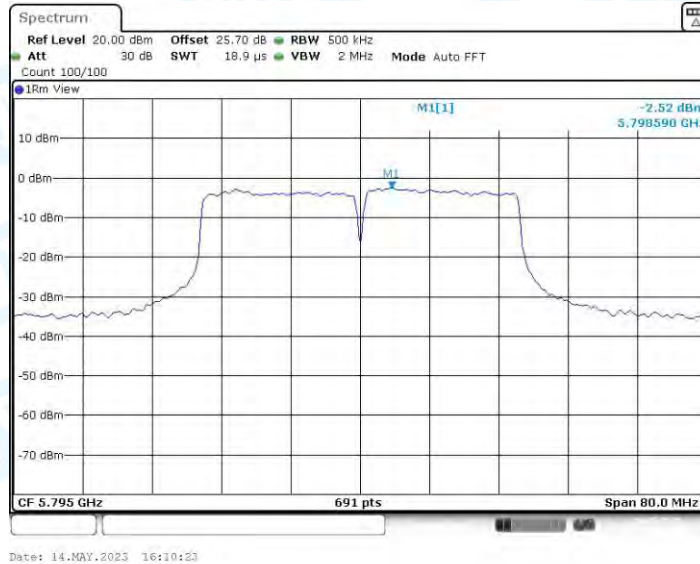
11AC40MIMO_Ant3_5795
