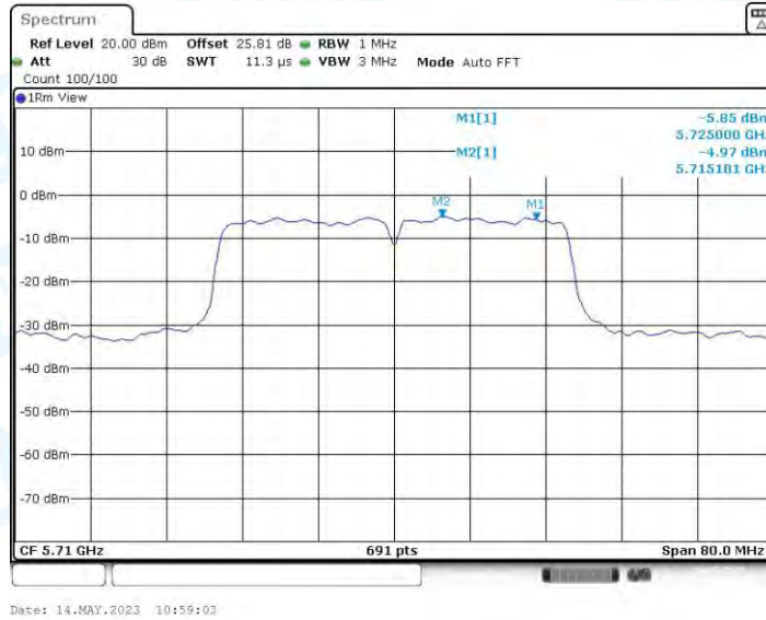
11N40MIMO_Ant3_5710_UNII-2C
