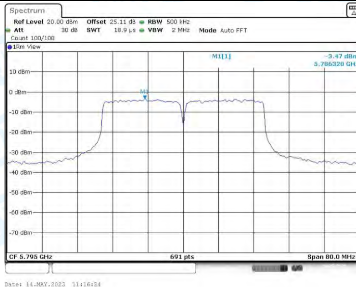
11N40MIMO_Ant4_5795
