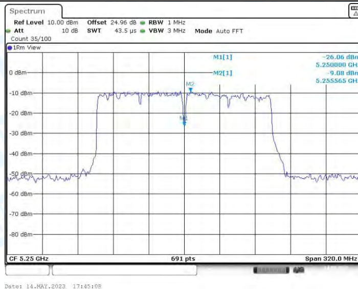
11AC160MIMO_Ant4_5250_UNII-2A
