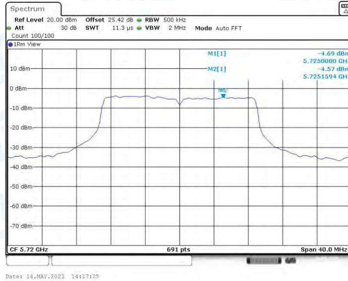
11AC20MIMO_Ant4_5720_UNII-3
