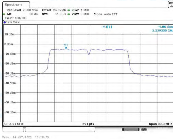
11N40MIMO_Ant4_5270
