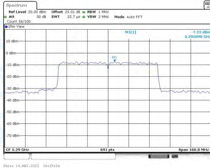
11AC80MIMO_Ant4_5290
