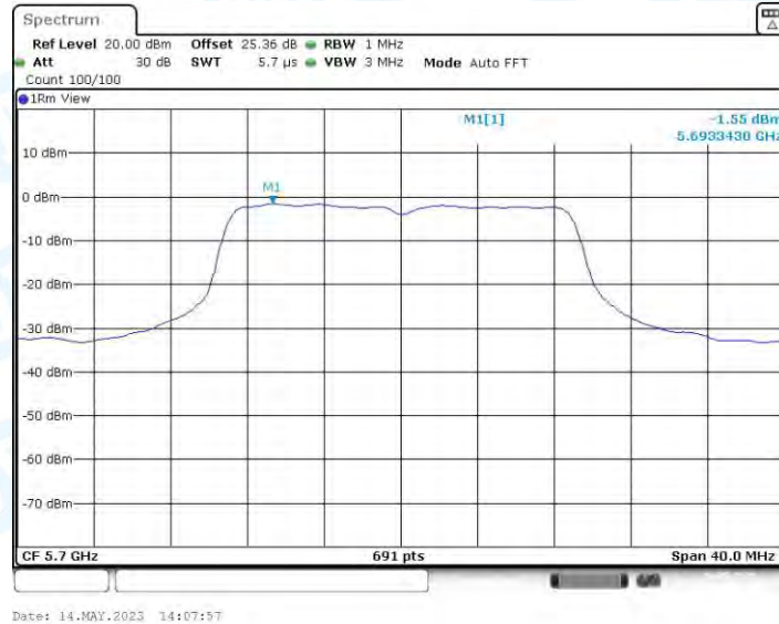
11AC20MIMO_Ant4_5700
