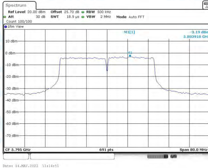
11N40MIMO_Ant3_5795
