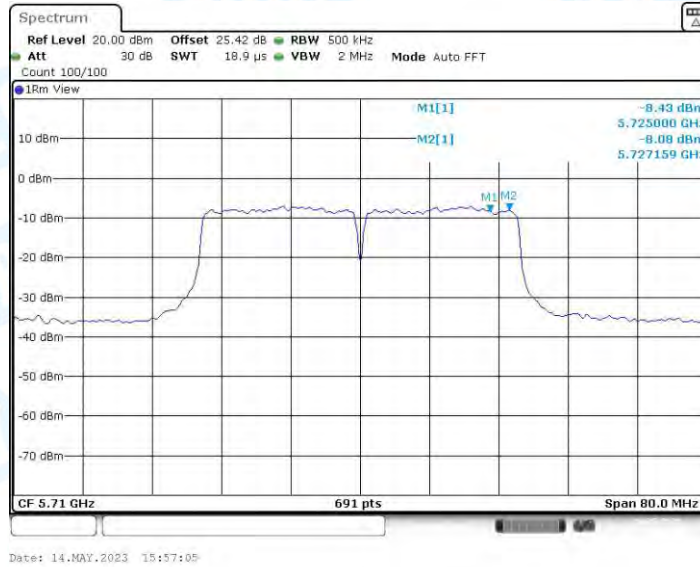
11AC40MIMO_Ant4_5710_UNII-3
