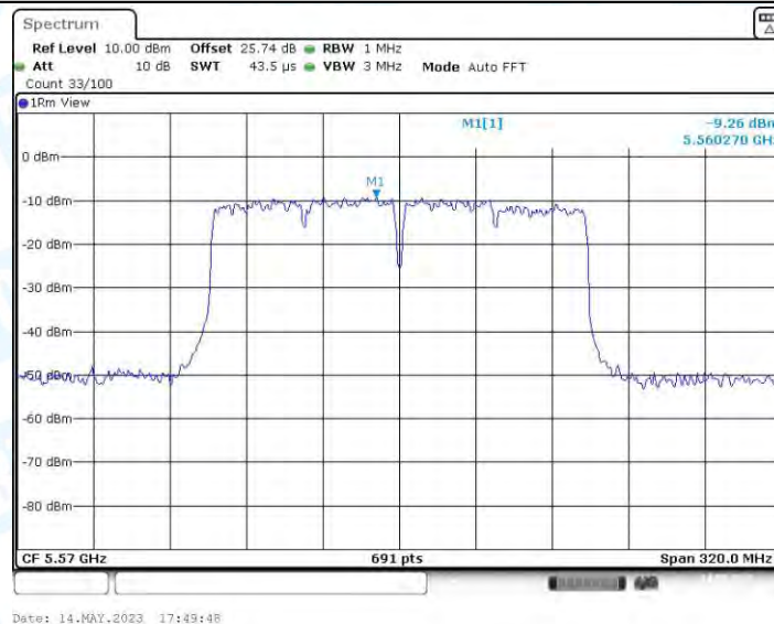
11AC160MIMO_Ant3_5570
