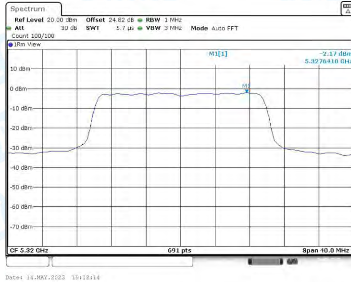
11AX20MIMO_Ant4_5320
