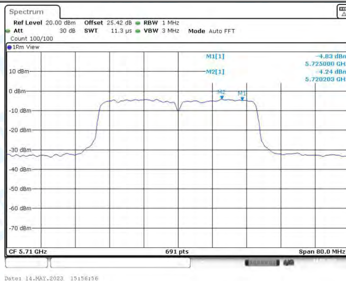
11AC40MIMO_Ant4_5710_UNII-2C
