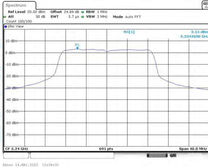
11AC20MIMO_Ant4_5240
