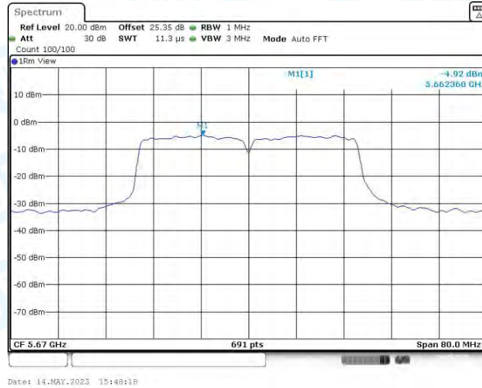
11AC40MIMO_Ant4_5670
