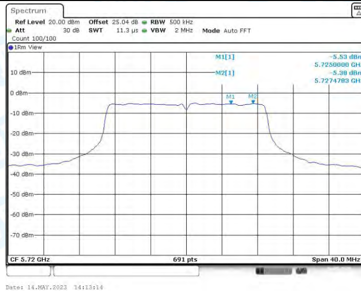
11AC20MIMO_Ant2_5720_UNII-3
