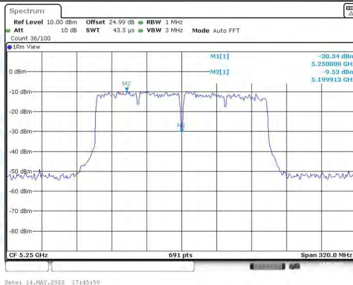
11AC160MIMO_Ant1_5250_UNII-2A
