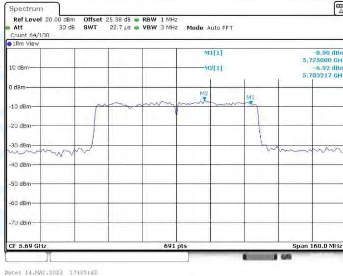
11AC80MIMO_Ant4_5690_UNII-2C
