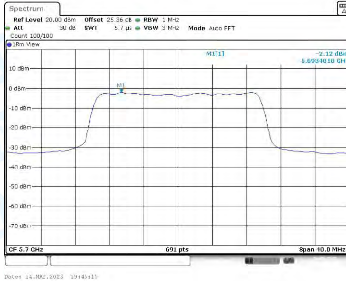
11AX20MIMO_Ant4_5700
