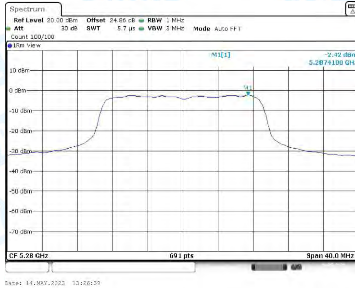
11AC20MIMO_Ant4_5280
