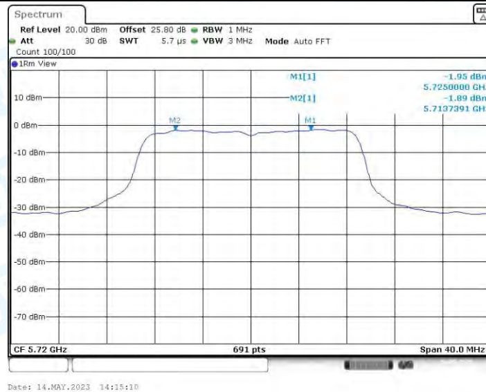
11AC20MIMO_Ant3_5720_UNII-2C
