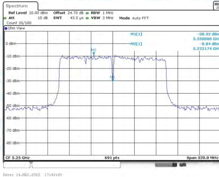
11AC160MIMO_Ant2_5250_UNII-1
