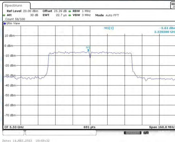
11AC80MIMO_Ant4_5530
