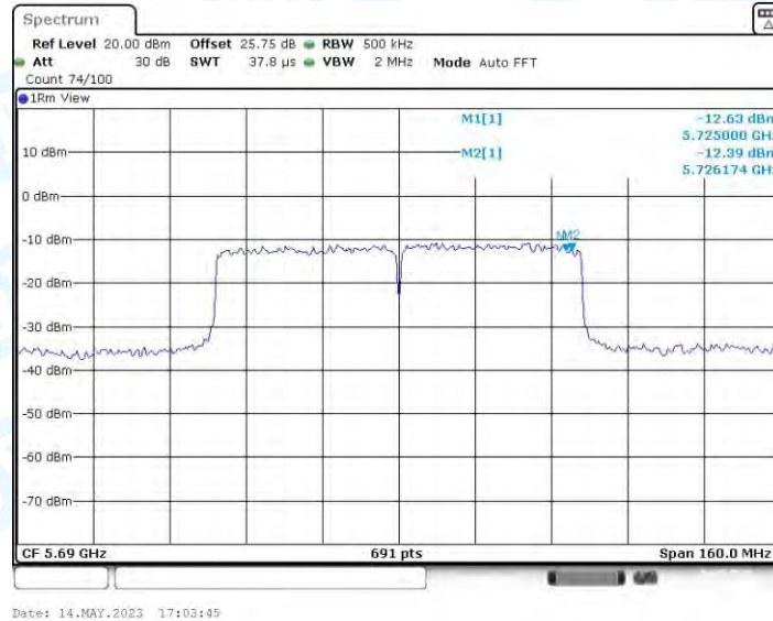
11AC80MIMO_Ant3_5690_UNII-3
