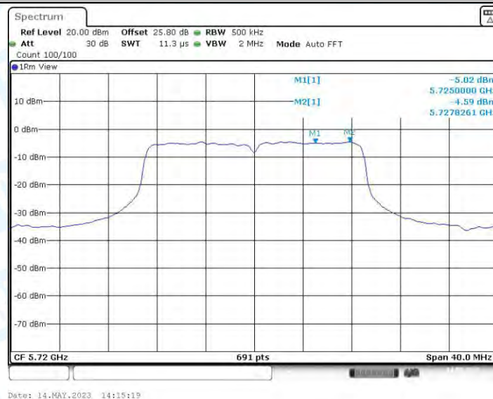
11AC20MIMO_Ant3_5720_UNII-3
