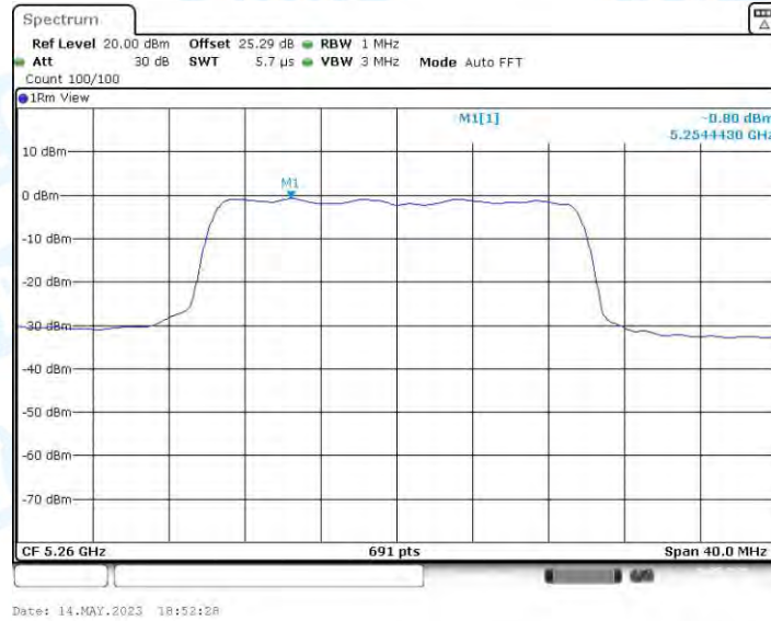
11AX20MIMO_Ant3_5260
