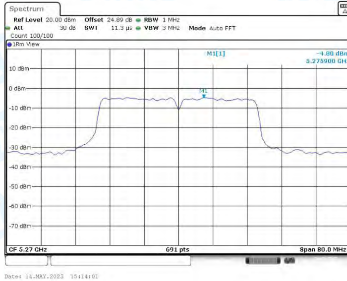
11AC40MIMO_Ant4_5270
