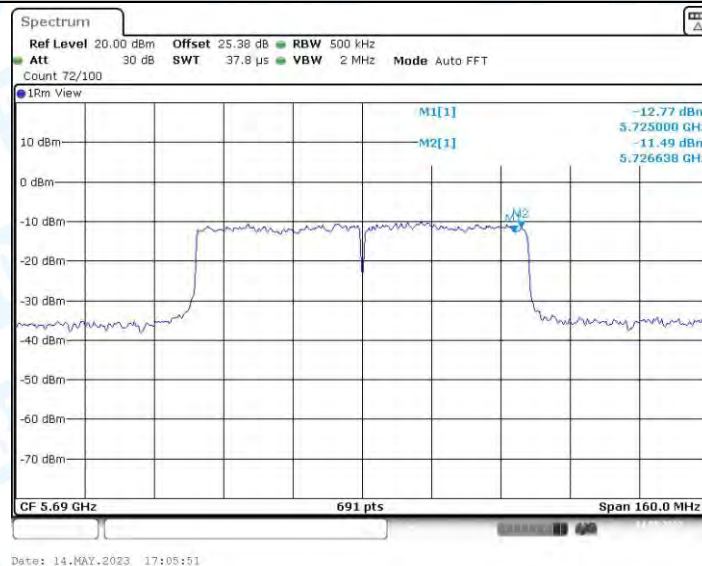
11AC80MIMO_Ant4_5690_UNII-3
