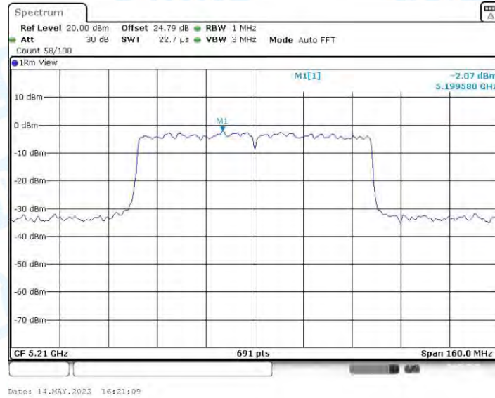
11AC80MIMO_Ant4_5210
