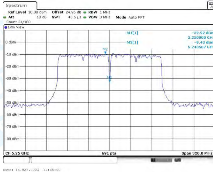
11AC160MIMO_Ant4_5250_UNII-1
