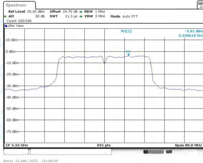
11AC40MIMO_Ant2_5550
