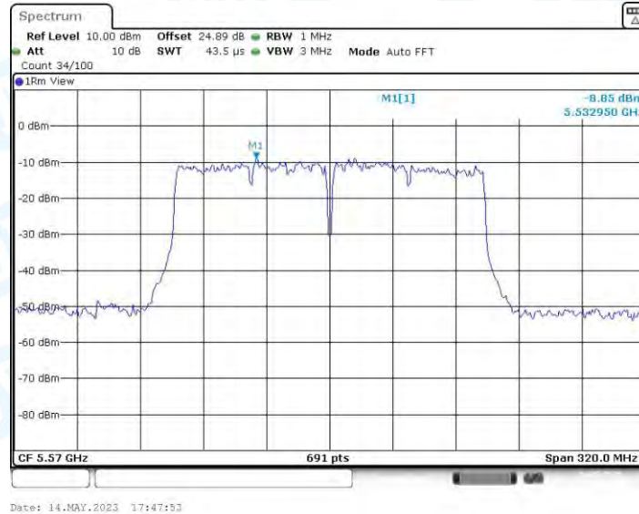
11AC160MIMO_Ant2_5570
