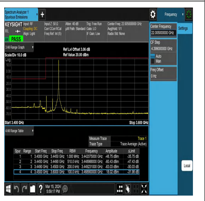
Band42_20MHz_QPSK_42190_1RB#99
