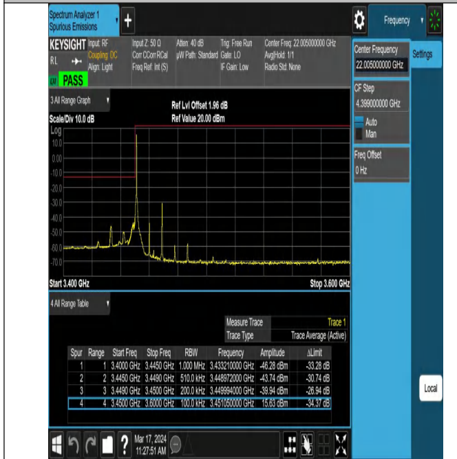
Band42_20MHz_QPSK_42190_1RB#0
