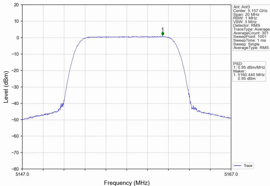
10_LCH_5157MHz_Ant3_NTNV
