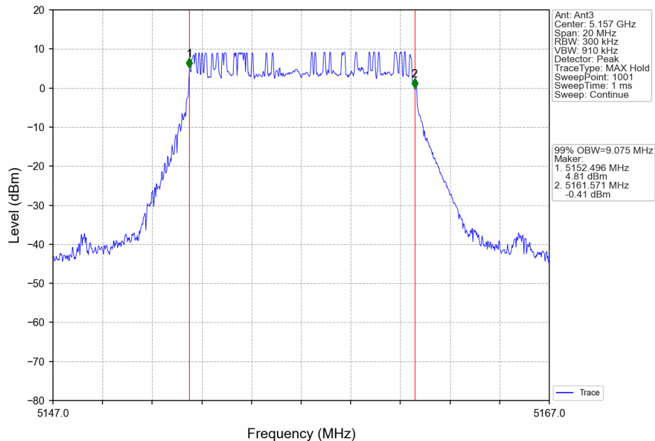
10_LCH_5157MHz_Ant3_NTNV
