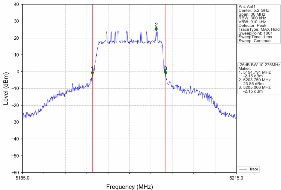
10_MCH_5200MHz_Ant1_NTNV
