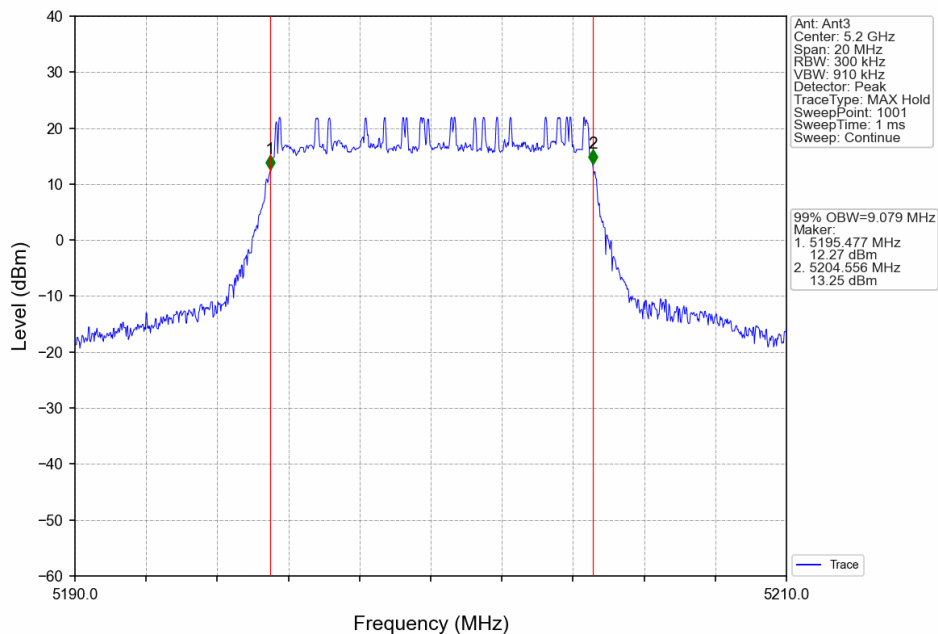
10_MCH_5200MHz_Ant3_NTNV
