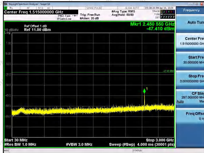
11AX80SISO-Ant1-6705-30~3000-PASS
