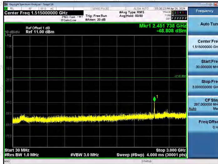
11AX80SISO-Ant1-6545-30~3000-PASS
