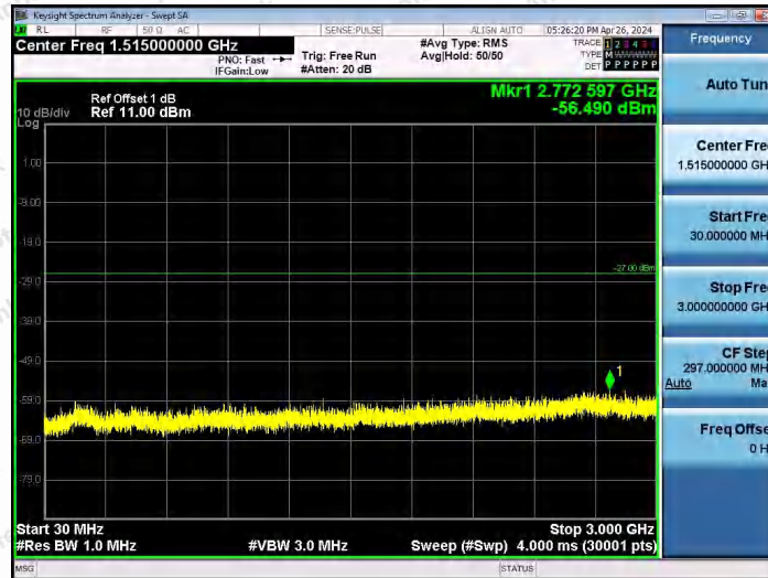
11AX80SISO-Ant1-6385-30~3000-PASS
