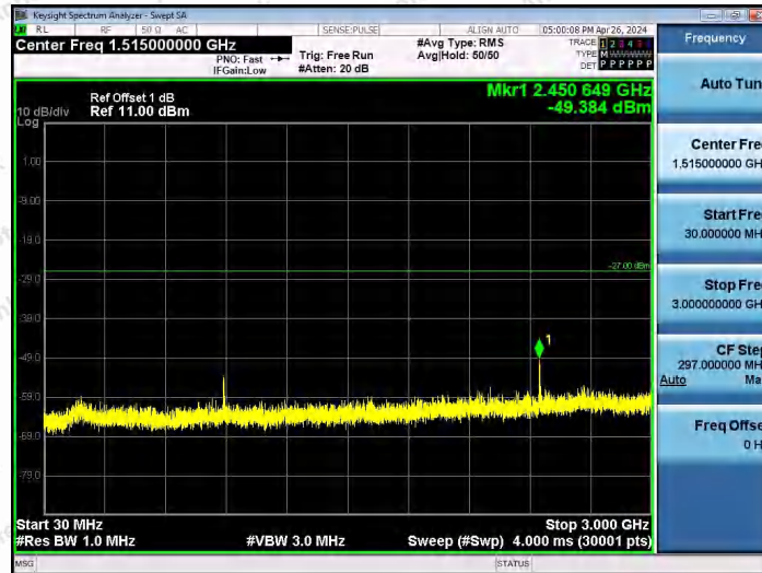
11AX40SISO-Ant1-6405-30~3000-PASS
