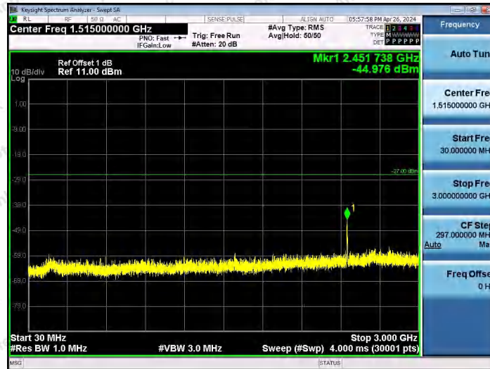
11AX80SISO-Ant1-6945-30~3000-PASS
