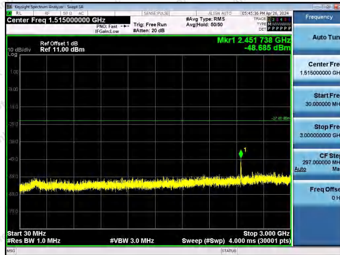
11AX80SISO-Ant1-6865-30~3000-PASS
