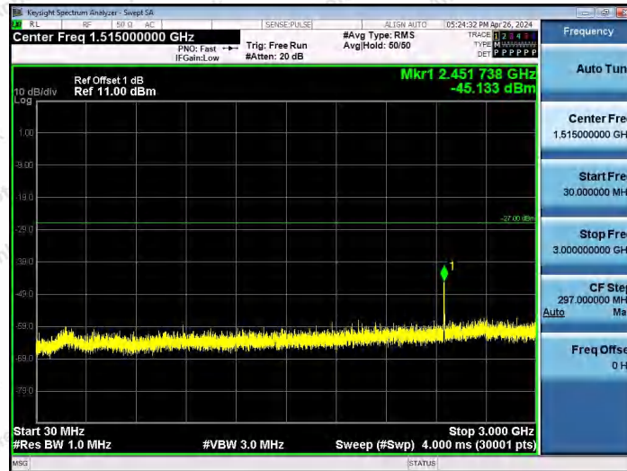
11AX80SISO-Ant1-6145-30~3000-PASS
