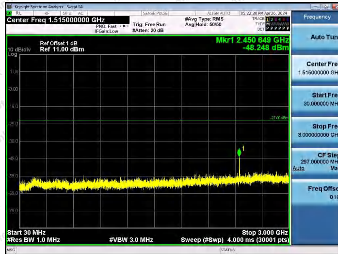
11AX80SISO-Ant1-5985-30~3000-PASS
