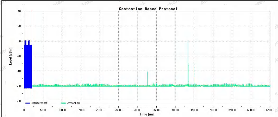
11AX80SISO-Ant1-5985-5985-PASS
