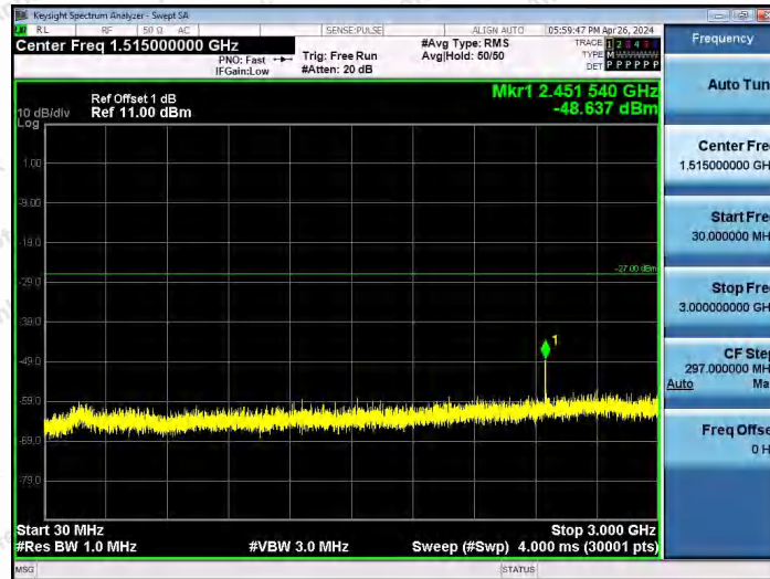
11AX80SISO-Ant1-7025-30~3000-PASS
