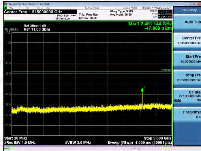
11AX80SISO-Ant1-6465-30~3000-PASS
