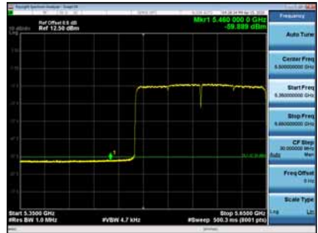
5570MHz with 4*4 Beamforming AV
