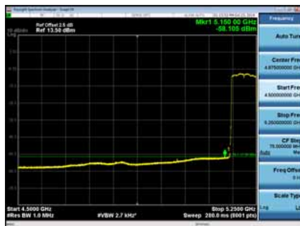
5210MHz with 4*4 CDD AV
