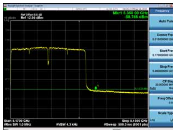
5250MHz with 4*4 Beamforming AV
