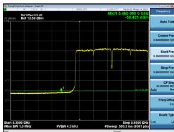
5570MHz with 4*4 CDD AV
