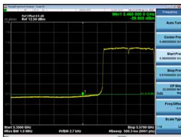
5530MHz with 4*4 CDD AV
