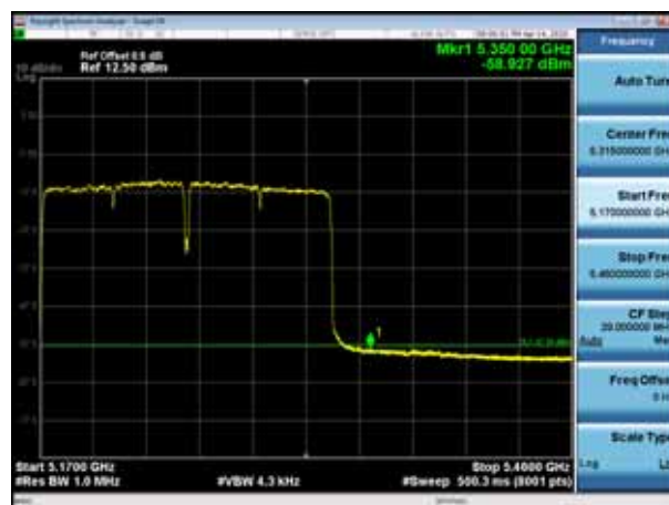
5250MHz with 4*4 CDD AV
