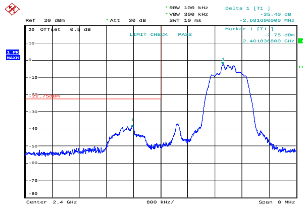
\pi/4 -DQPSK_Low 35.40 dB
