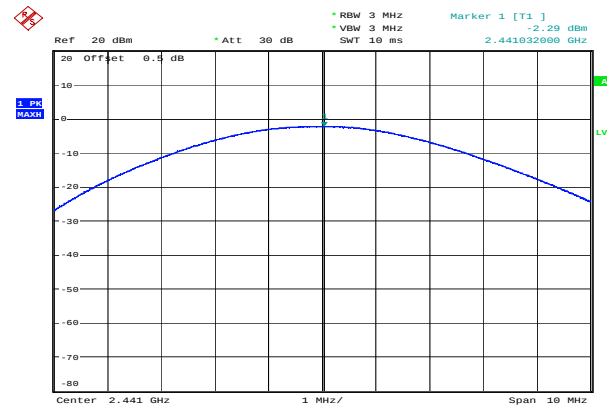
\pi/4 -DQPSK_Middle -2.29 dBm
