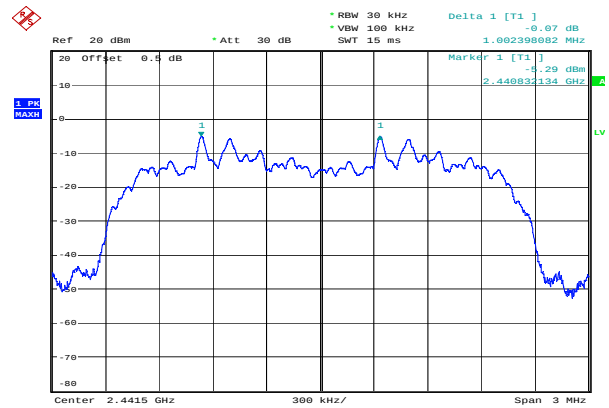
\pi/4 -DQPSK_Middle 1.002 MHz
