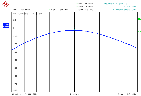
\pi/4 -DQPSK_High -3.05 dBm
