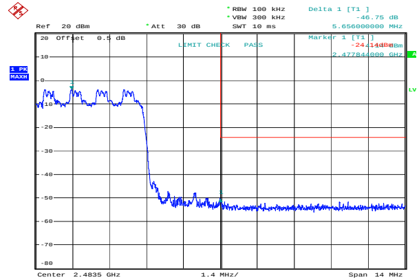
\pi/4 -DQPSK_Hopping_Upper 46.75 dB
