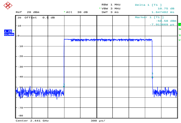
\pi/4 -DQPSK_Hopping_2DH3 1.647ms
