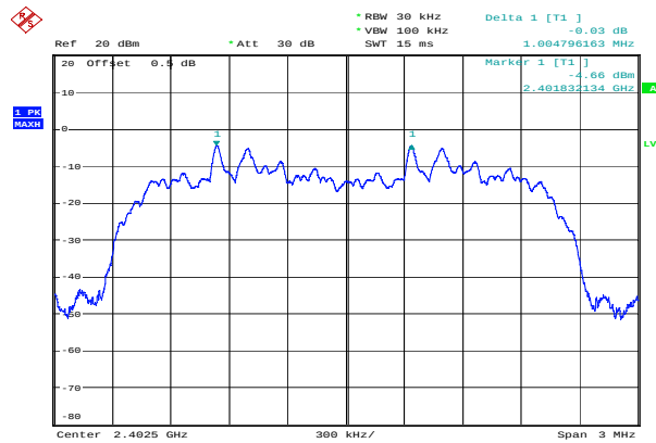
\pi/4 -DQPSK_Low 1.005 MHz
