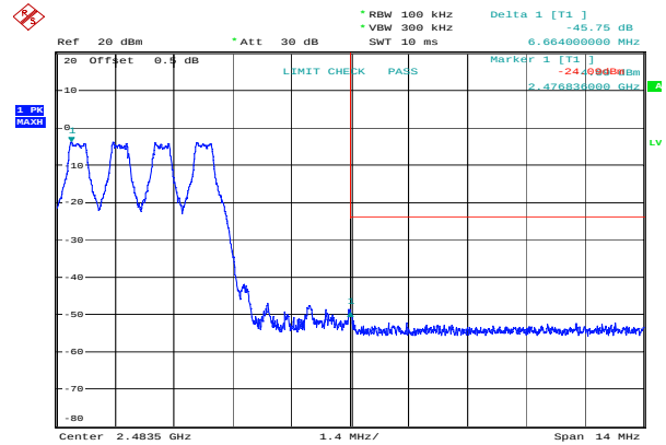
GFSK_Hopping_Upper 45.75 dB
