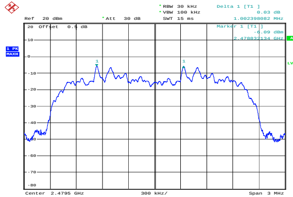
\pi/4 -DQPSK_High 1.002 MHz
