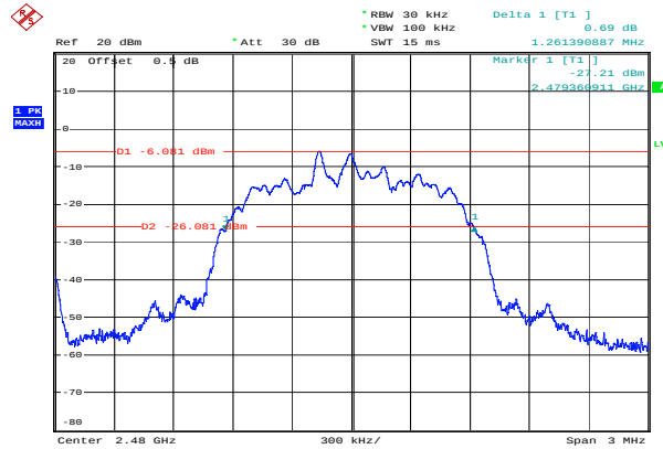
\pi/4 -DQPSK_High 1.261 MHz
