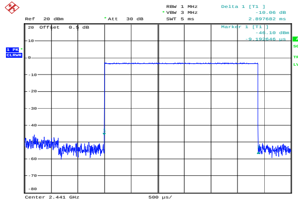
GFSK_Hopping_DH5 2.898ms
