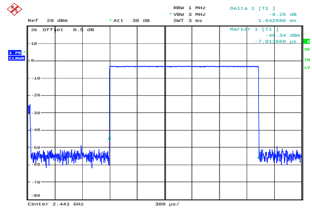
GFSK_Hopping_DH3 1.643ms
