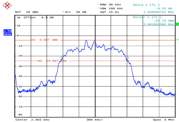
\pi/4 -DQPSK_Low 1.257 MHz
