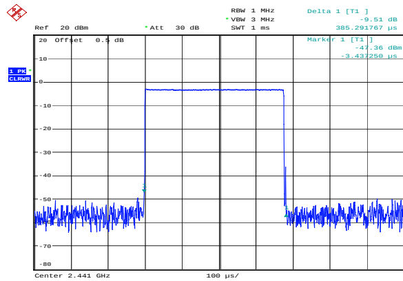
GFSK_Hopping_DH1 0.385ms
