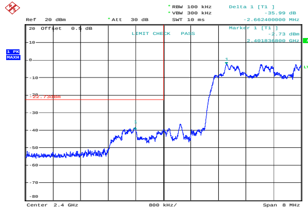
\pi/4 -DQPSK_Hopping_Lower 35.99 dB
