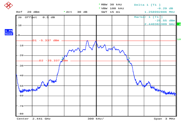
\pi/4 -DQPSK_Middle 1.259 MHz
