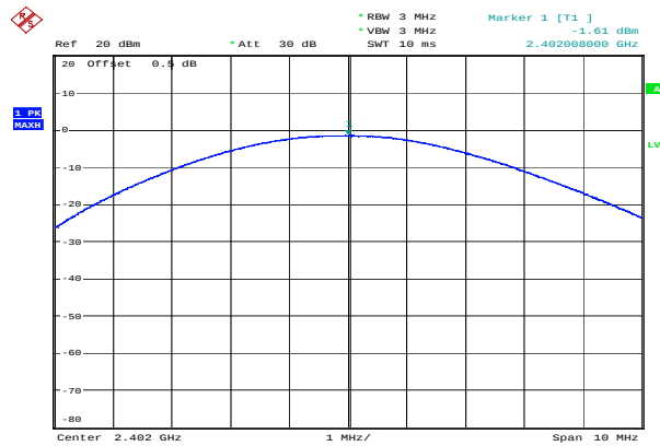
\pi/4 -DQPSK_Low -1.61 dBm
