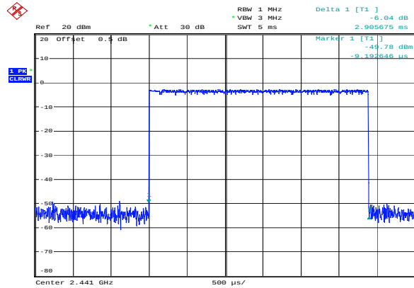
\pi/4 -DQPSK_Hopping_2DH5 2.906ms
