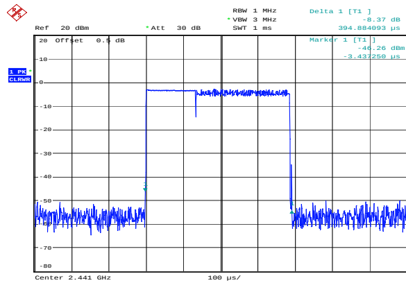
\pi/4 -DQPSK_Hopping_2DH1 0.395ms
