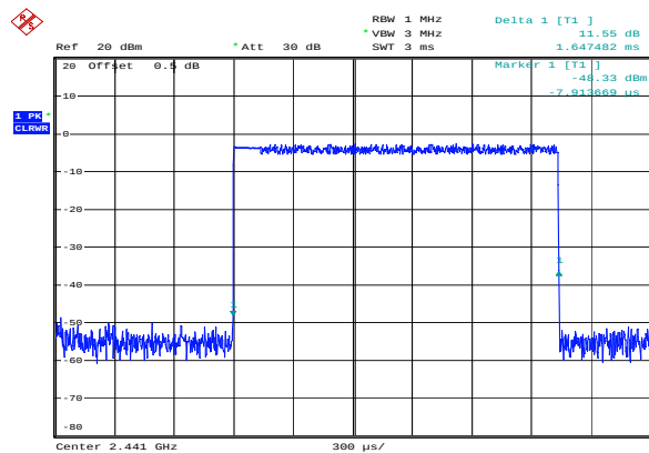
8DPSK_Hopping_3DH3 1.647ms
