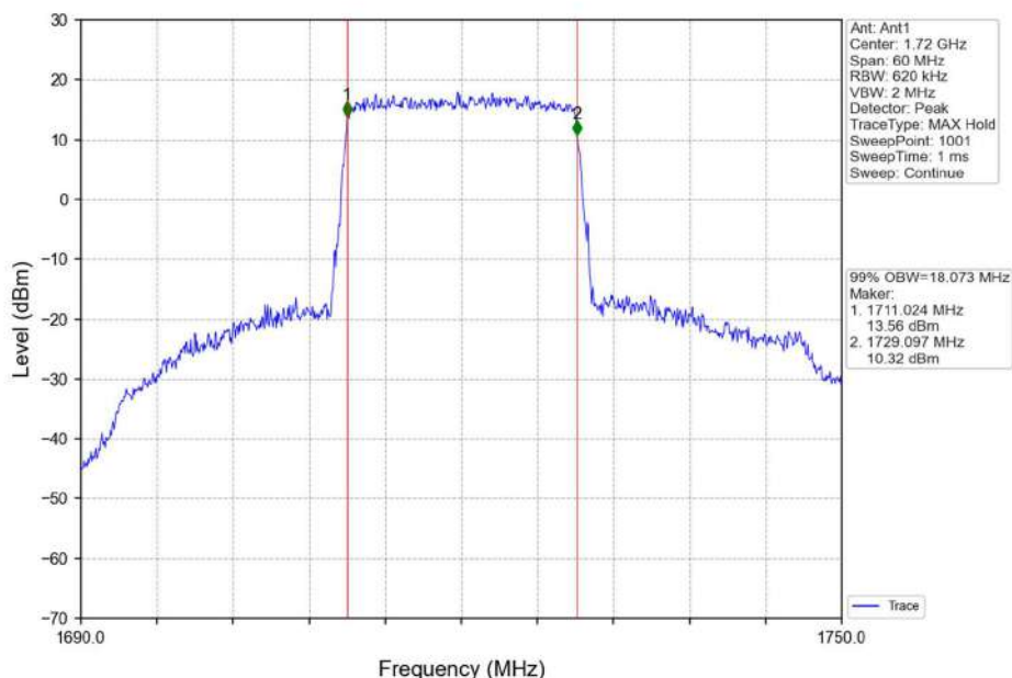
Band66_20MHz_QPSK_LCH_1720MHz_RB_100_0_NTNV
