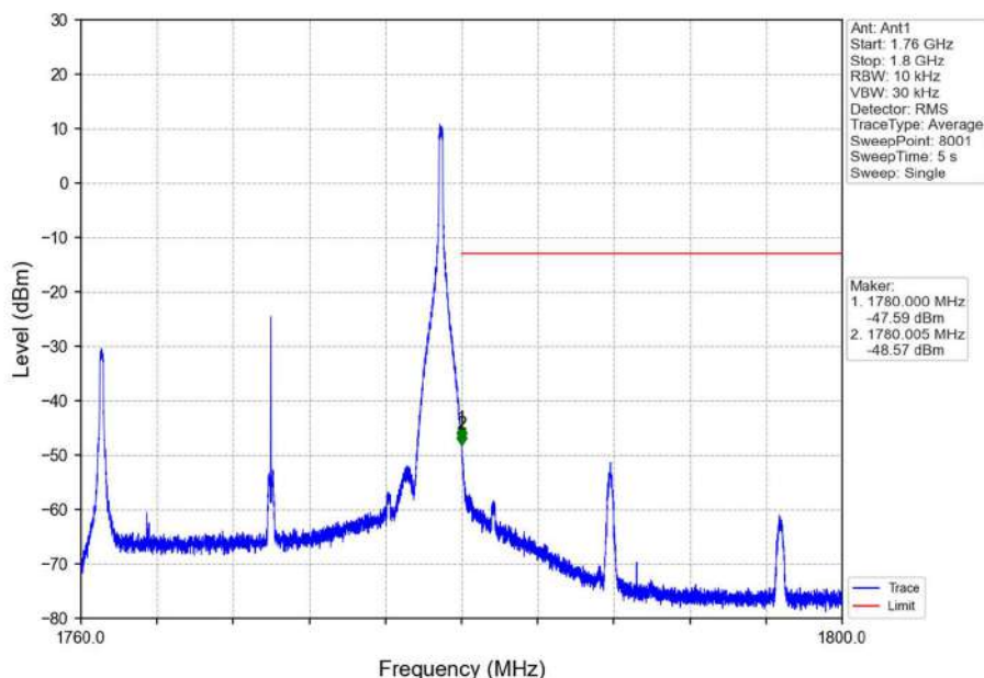
Band66_20MHz_QPSK_HCH_1770MHz_RB_1_99_NTNV
