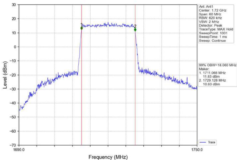
Band66_20MHz_16QAM_LCH_1720MHz_RB_100_0_NTNV
