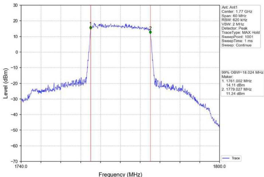
Band66_20MHz_QPSK_HCH_1770MHz_RB_100_0_NTNV
