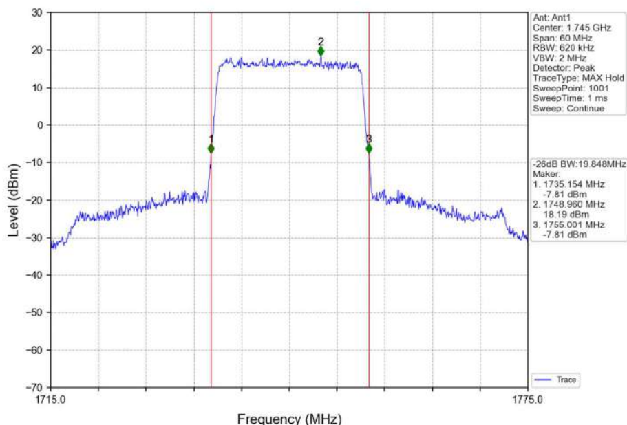
Band66_20MHz_QPSK_MCH_1745MHz_RB_100_0_NTNV
