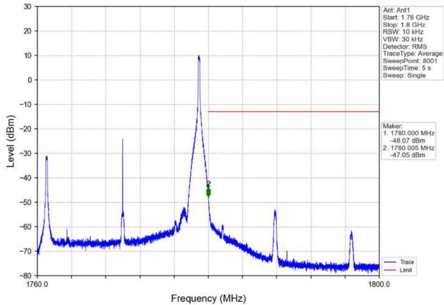
Band66_20MHz_16QAM_HCH_1770MHz_RB_1_99_NTNV
