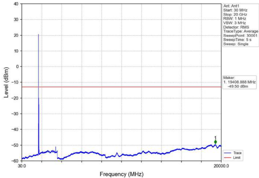
Band66_20MHz_16QAM_LCH_1720MHz_RB_1_0_NTNV
