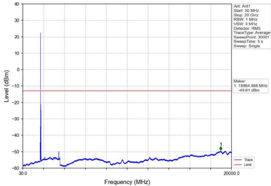
Band66_20MHz_QPSK_MCH_1745MHz_RB_1_0_NTNV
