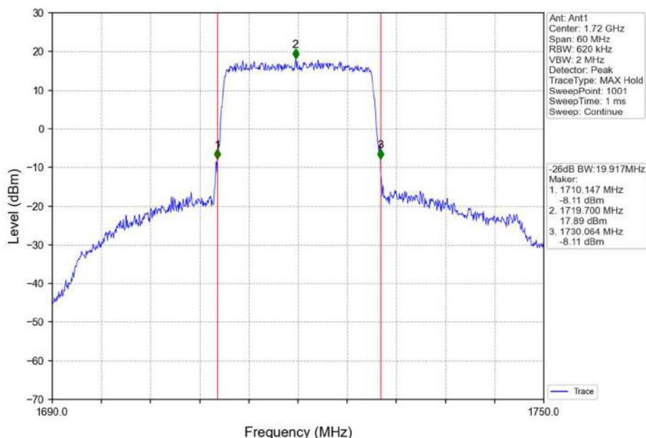
Band66_20MHz_QPSK_LCH_1720MHz_RB_100_0_NTNV
