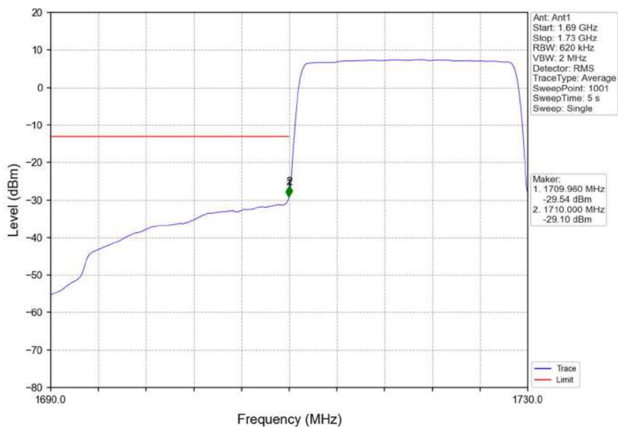
Band66_20MHz_QPSK_LCH_1720MHz_RB_100_0_NTNV
