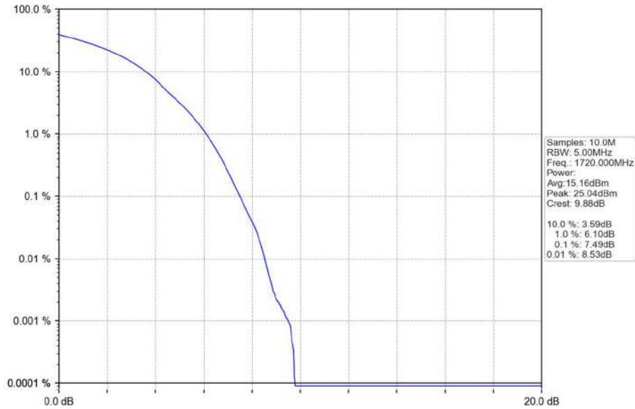
Band66_20MHz_16QAM_LCH_1720MHz_RB_100_0_NTNV
