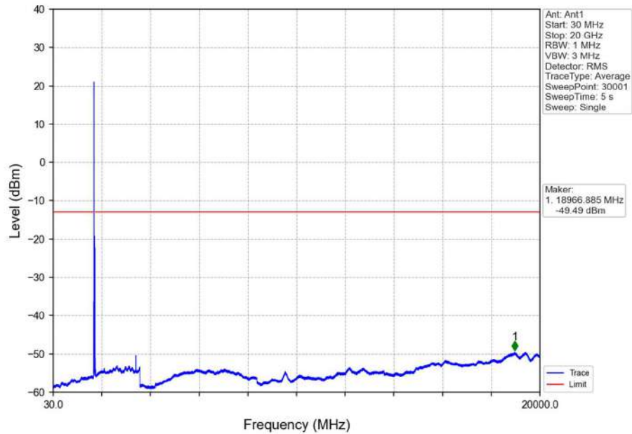
Band66_20MHz_QPSK_LCH_1720MHz_RB_1_0_NTNV
