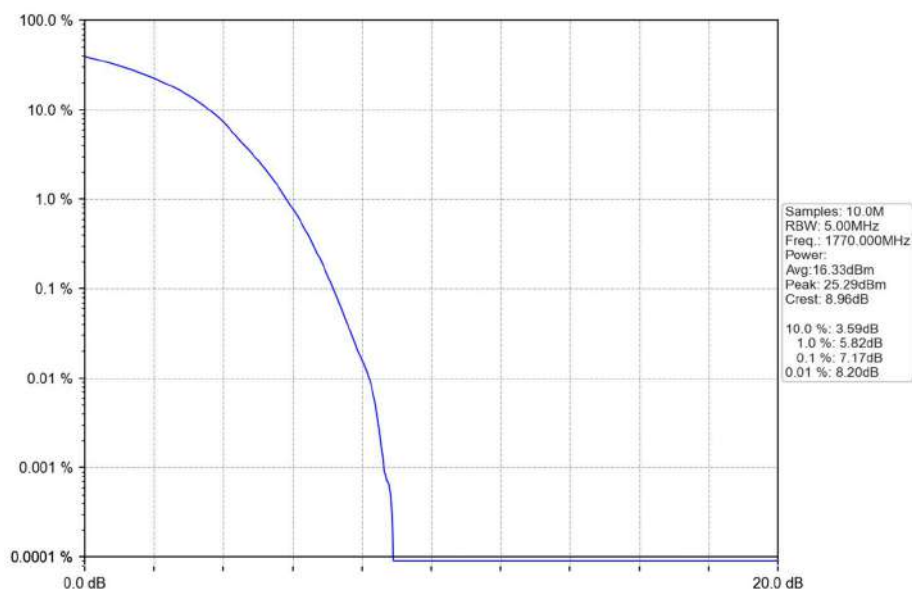
Band66_20MHz_QPSK_HCH_1770MHz_RB_100_0_NTNV
