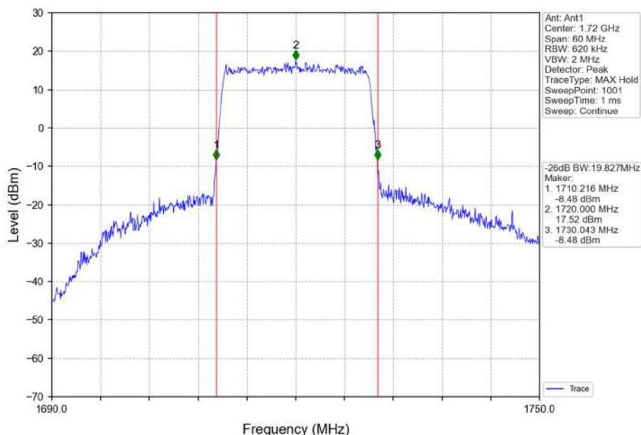
Band66_20MHz_16QAM_LCH_1720MHz_RB_100_0_NTNV
