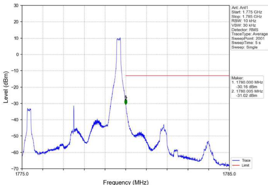
Band66_5MHz_QPSK_HCH_1777.5MHz_RB_1_24_NTNV
