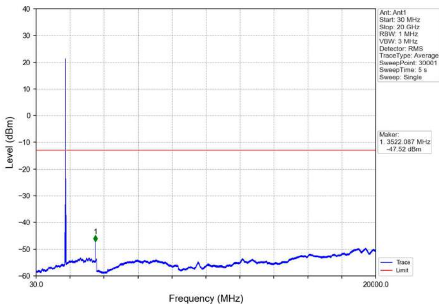
Band66_20MHz_QPSK_HCH_1770MHz_RB_1_0_NTNV
