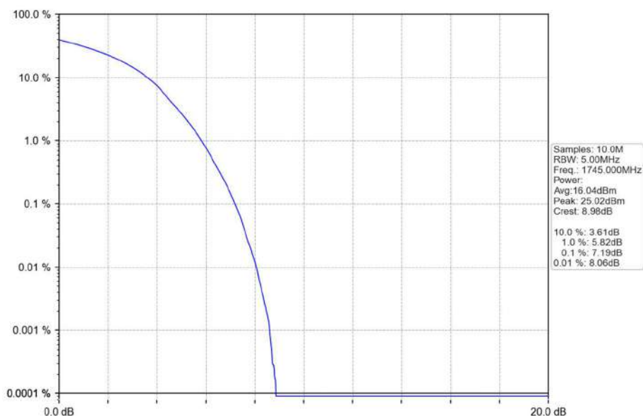
Band66_20MHz_QPSK_MCH_1745MHz_RB_100_0_NTNV
