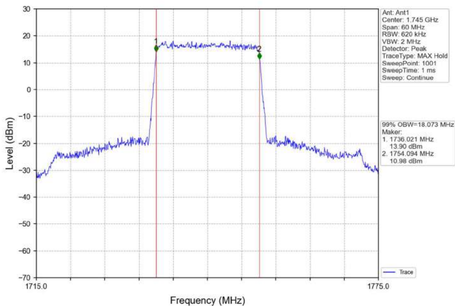
Band66_20MHz_QPSK_MCH_1745MHz_RB_100_0_NTNV
