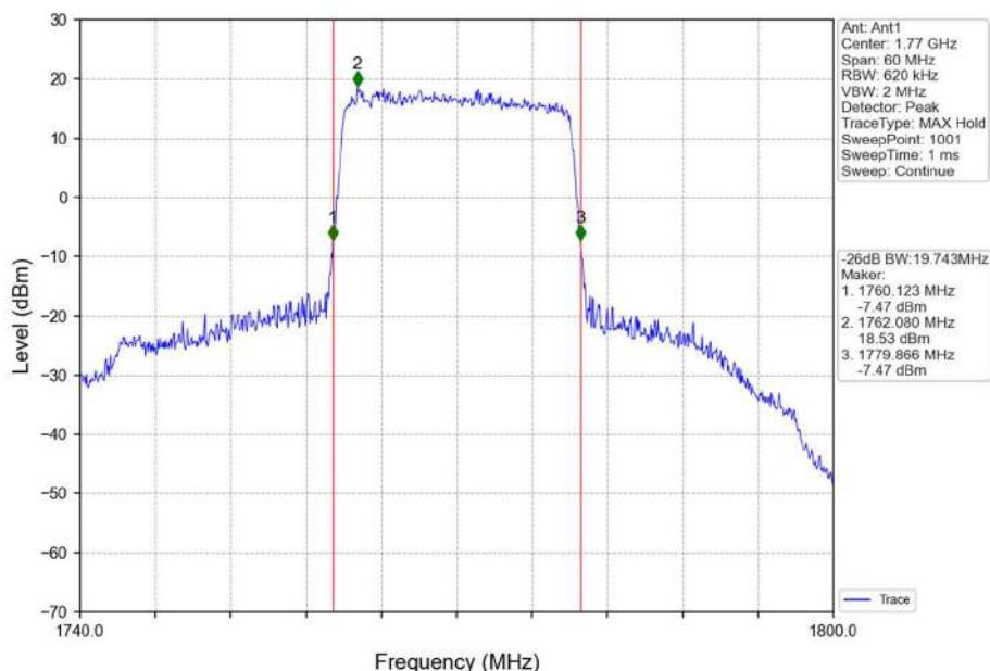
Band66_20MHz_QPSK_HCH_1770MHz_RB_100_0_NTNV
