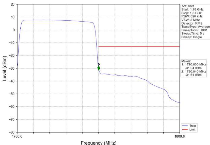
Band66_20MHz_QPSK_HCH_1770MHz_RB_100_0_NTNV
