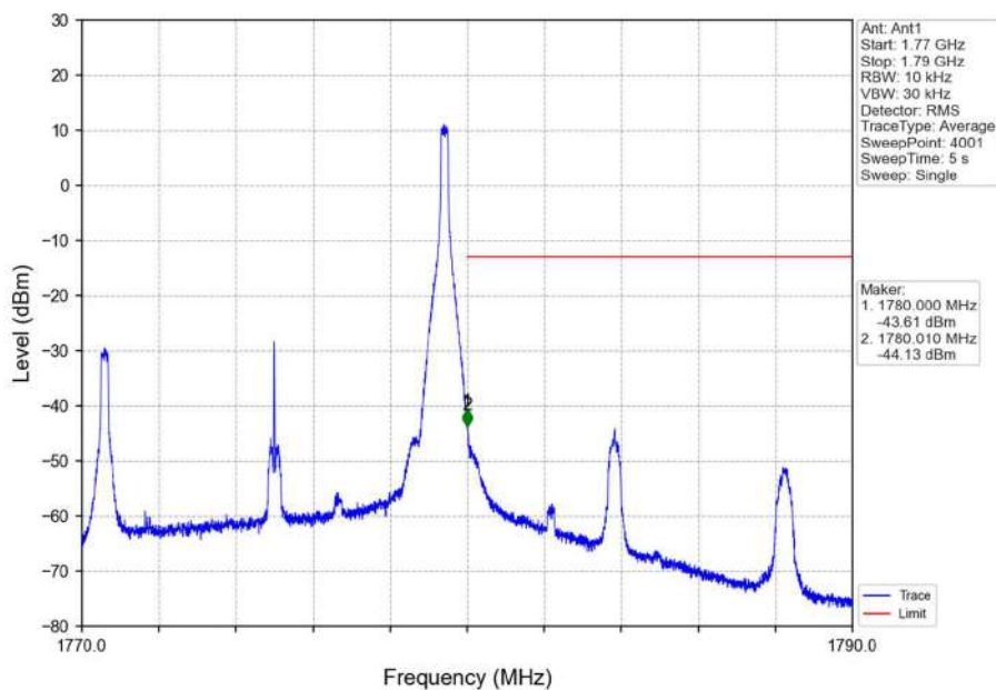
Band66_10MHz_QPSK_HCH_1775MHz_RB_1_49_NTNV
