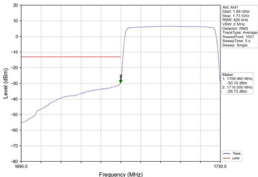
Band66_20MHz_16QAM_LCH_1720MHz_RB_100_0_NTNV
