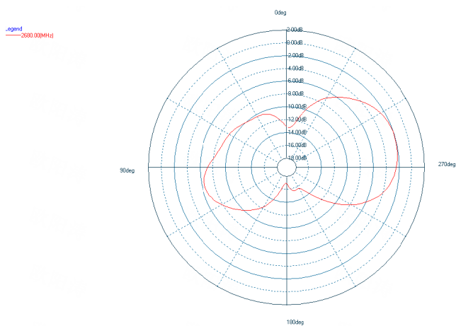
LTE B7/38/41 Phi=90deg
