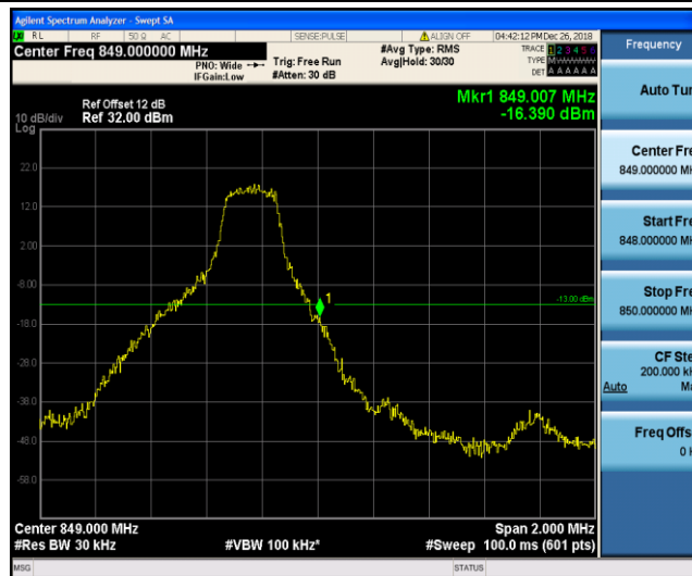
Band5_3MHz_QPSK_20635_1RB#14
