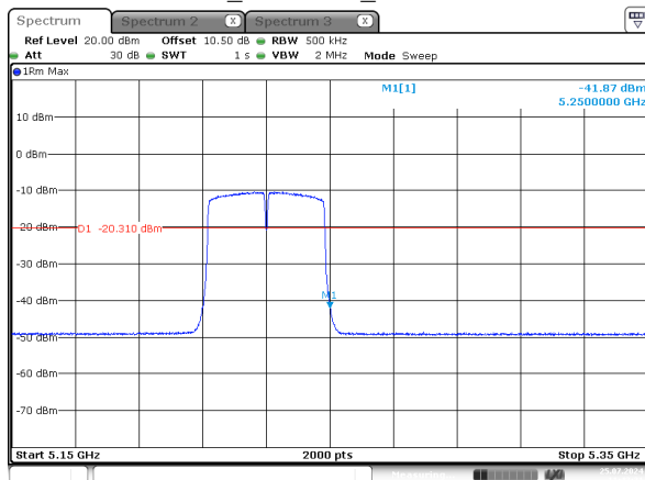
n40_5230MHz_Chain 2
