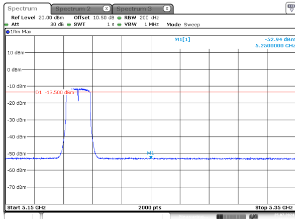
a_5200MHz_Chain 2
