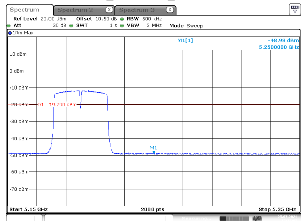
n40_5230MHz_Chain 3
