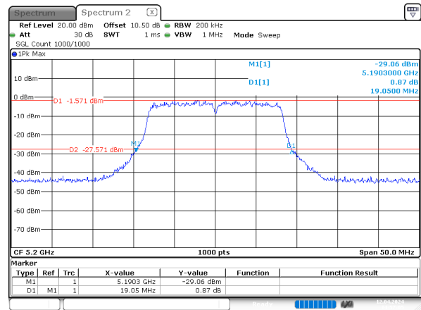
a_5200MHz_Chain 0
