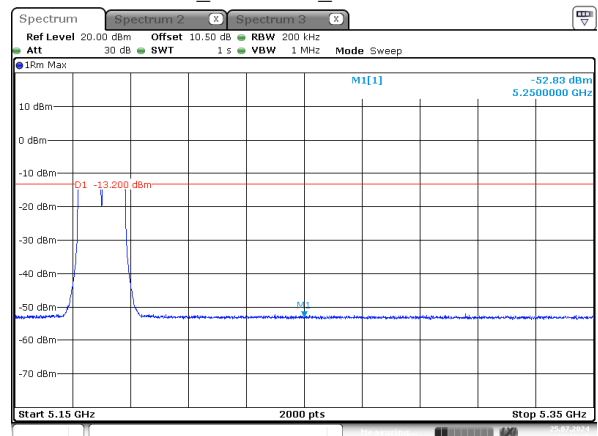
a_5180MHz_Chain 3
