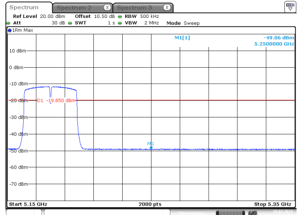
n40_5190MHz_Chain 3
