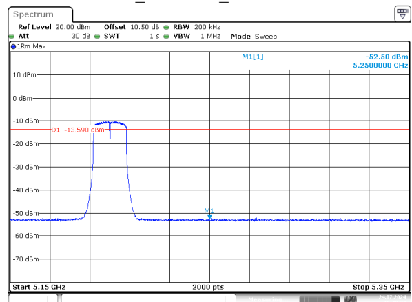
a_5200MHz_Chain 1
