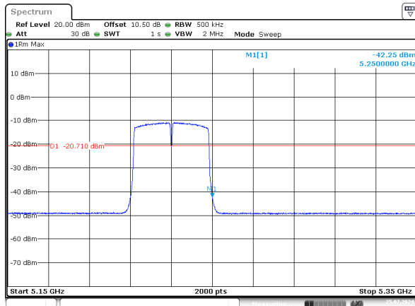
n40_5230MHz_Chain 0
