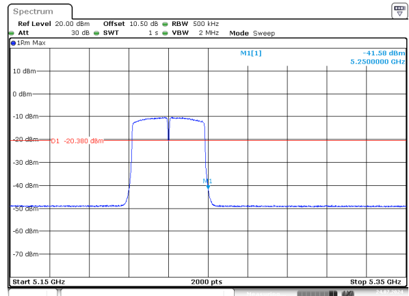
n40_5230MHz_Chain 1
