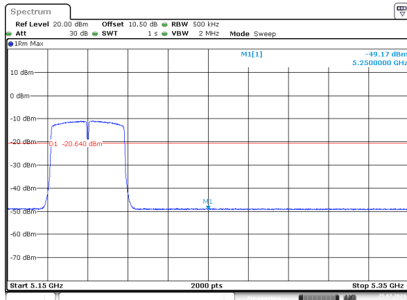
n40_5190MHz_Chain 0
