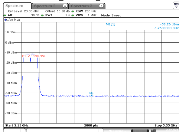
a_5180MHz_Chain 2
