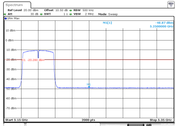
n40_5190MHz_Chain 1
