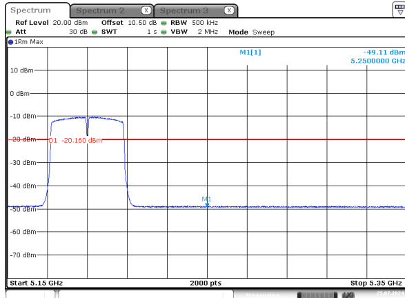
n40_5190MHz_Chain 2
