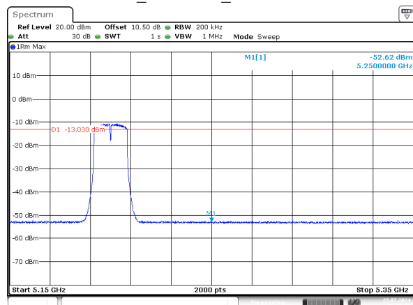
a_5200MHz_Chain 0
