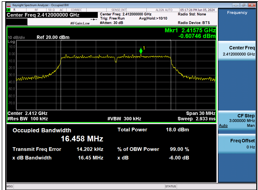
Test_Graph_802.11g_ANT1_2412_6Mbps_DTBSW
