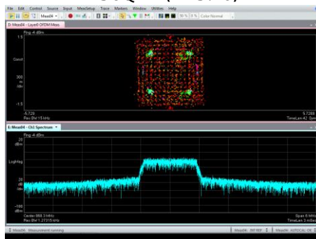
256QAM (TM3.1a)
