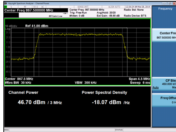
Ch_Power_TM3.1a_1C_3MBW_867_TX1
