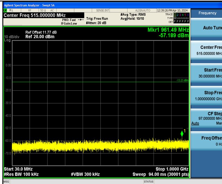
BLE_2M-Ant1-2440-30~1000-PASS
