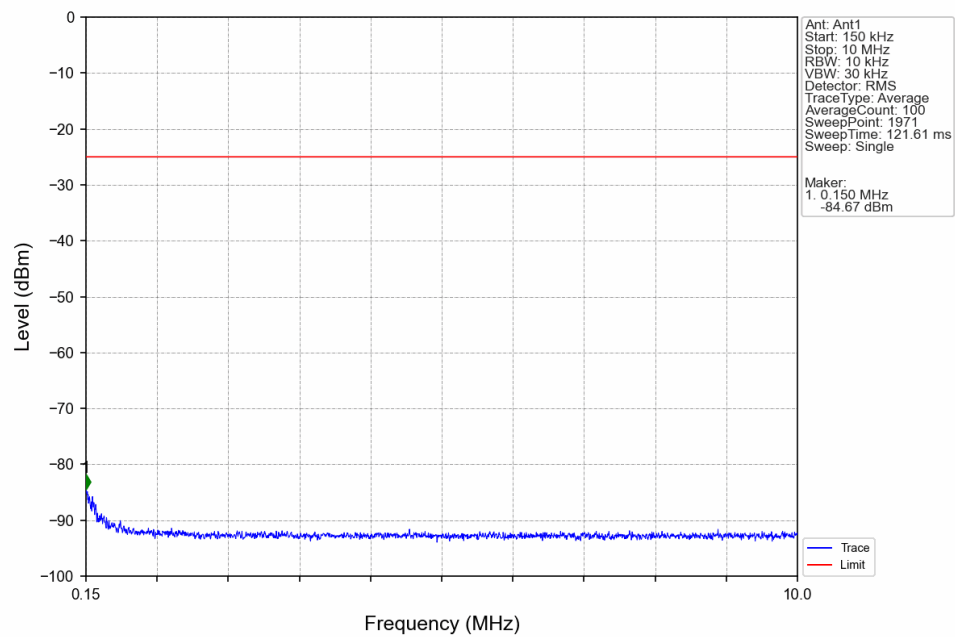
Band41_10MHz_16QAM_MCH_2593MHz_RB_1_0_NTNV
