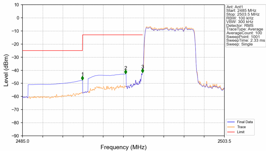
Band41_5MHz_QPSK_LCH_2498.5MHz_RB_25_0_NTNV
