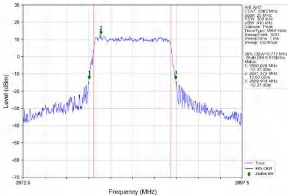
n41_30kHz_SISO_NTNV_10MHz_CP-OFDM_256_QAM_2685MHz_Outer_Full_Ant1
