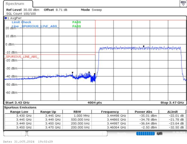
n77(3450-3550) SCS=30kHz DFT_16QAM BW=20MHz LowChannel=630668 RB=50@0
