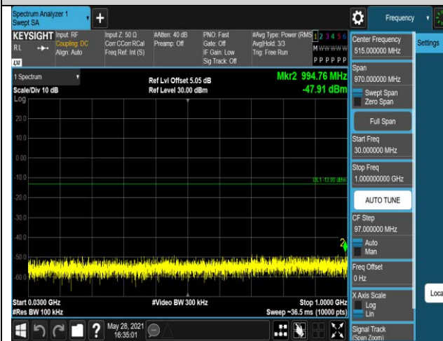
Band13-5MHz-QPSK-23205-1RB#0-Range1:30~10 00MHz
