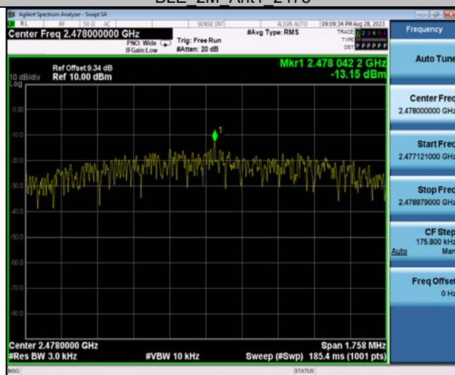
BLE 2M Ant1 2478
