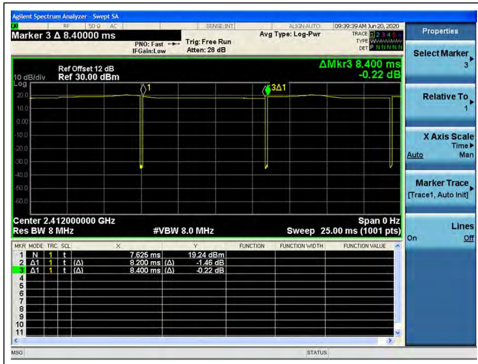
(Channel 1, 802.11b)
