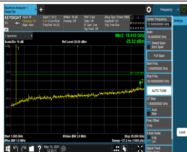
Band66-1.4MHz-QPSK-132665-1RB#0-Range2:1000~ 20000MHz
