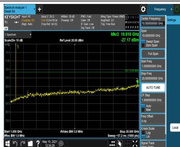
Band66-20MHz-QPSK-132072-1RB#0-Range2:1000~2
