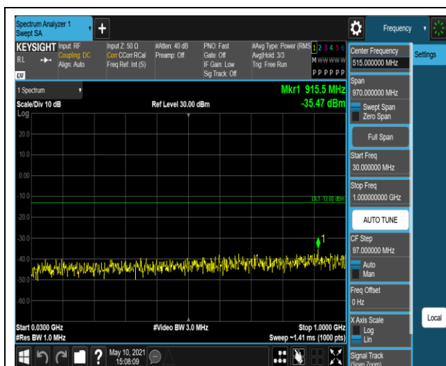
Band66-20MHz-QPSK-132572-1RB#0-Range1:30~1000MHz
