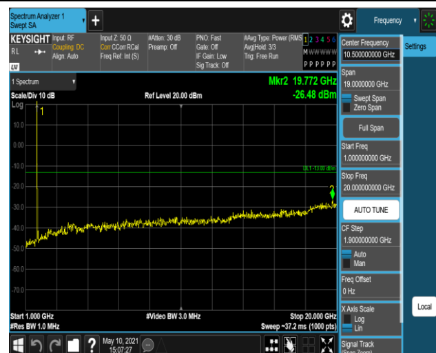
Band66-20MHz-QPSK-132322-1RB#0-Range2:1000~2
