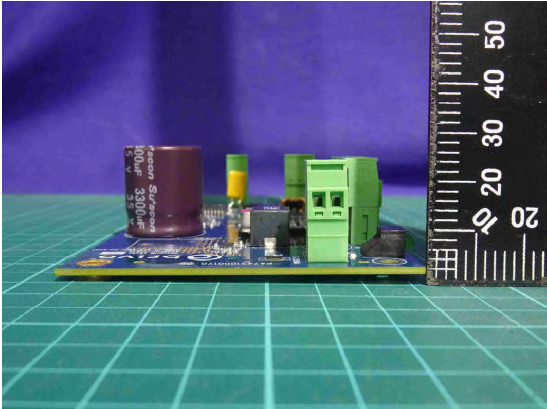
(158) EUT Photo
