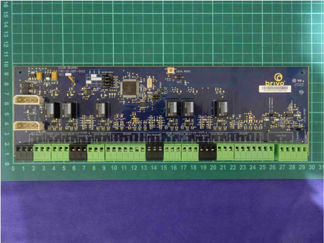
(144) EUT Photo
