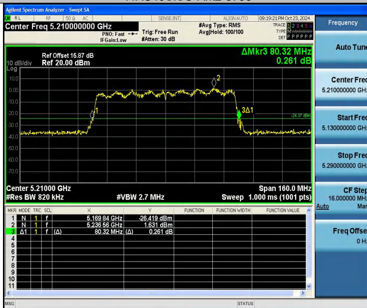
11AC80SISO-Ant2-5210
