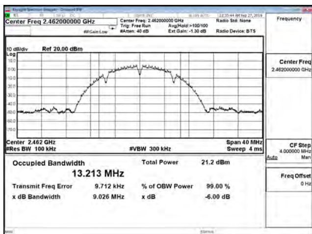
802.11b / Ant. 1 / 2462 MHz
