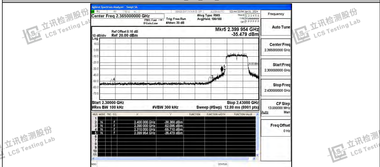
11N20SISO_Ant_Low_2412
