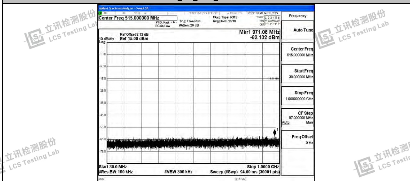
11B_Ant_2462_30~1000
