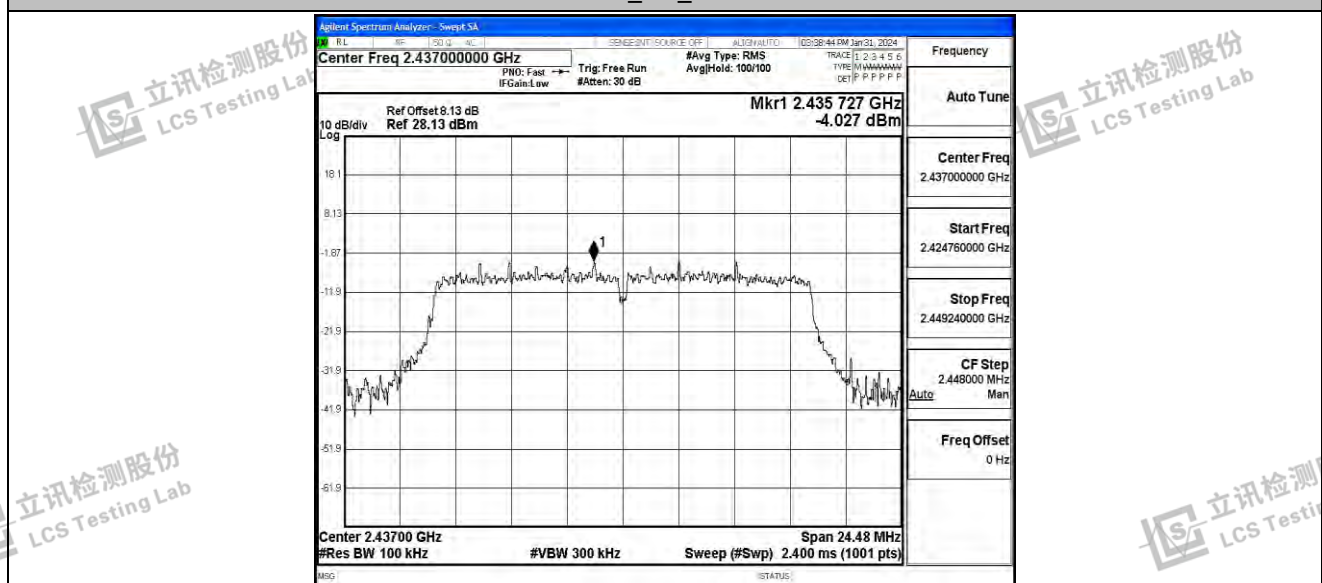
11G_Ant_2437
