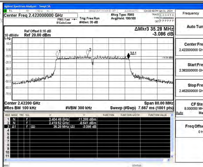
11N40ISO_Ant_2422
