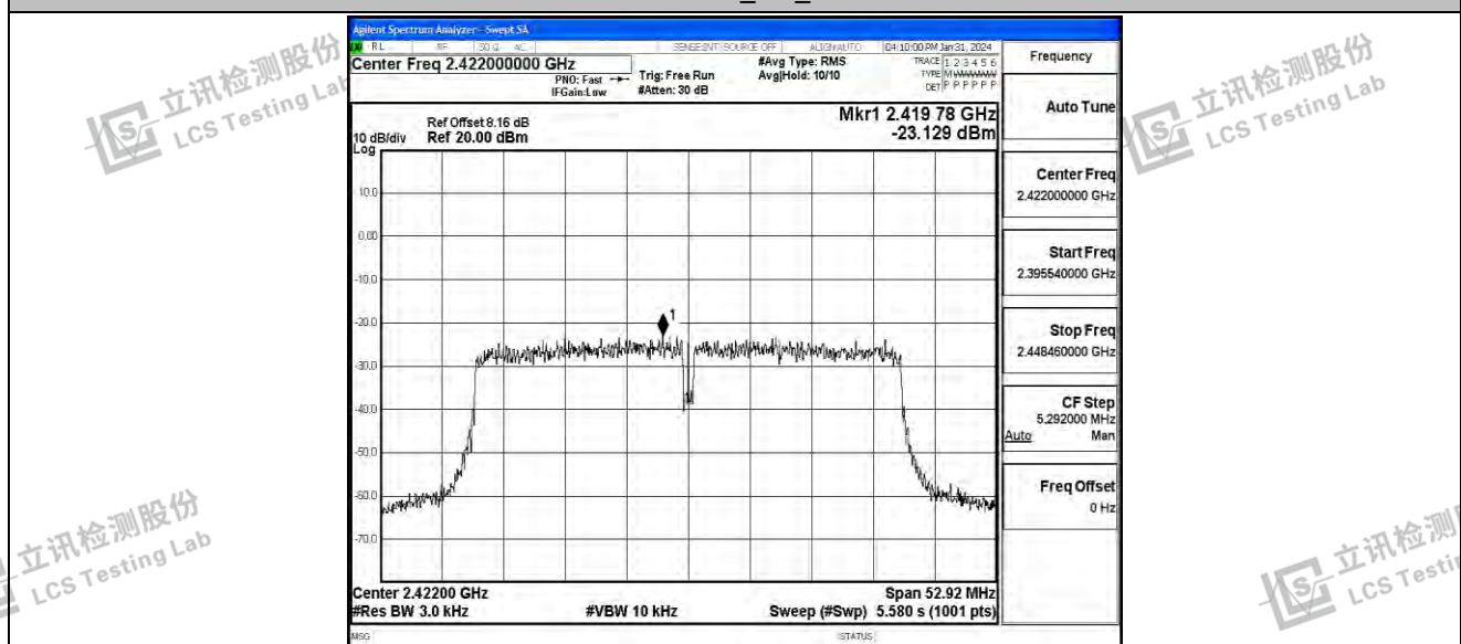
11N40SISO_Ant_2422
