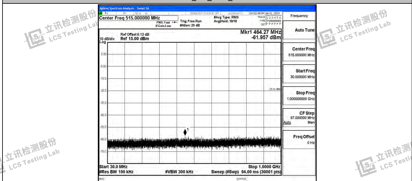
11N20SISO_Ant_2437_30~1000
