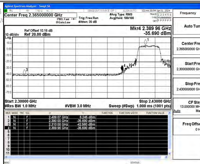
11N20ISO_Ant_Low_2412_Peak
