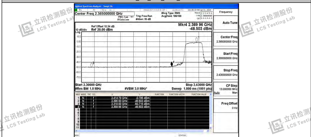
11G_Ant_Low_2412_AV
