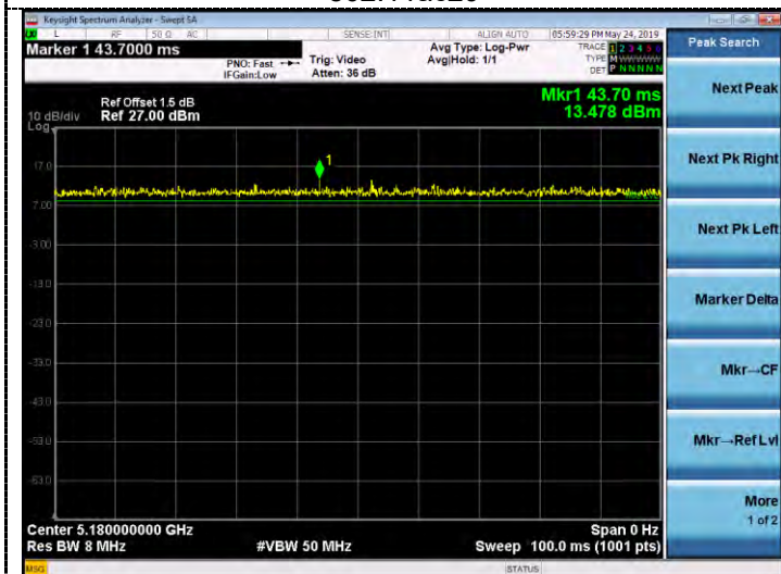
802.11ac20
