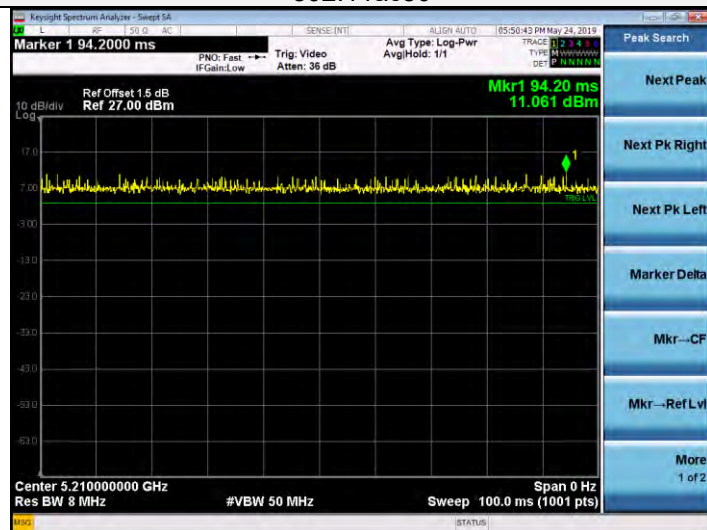
802.11ac80
