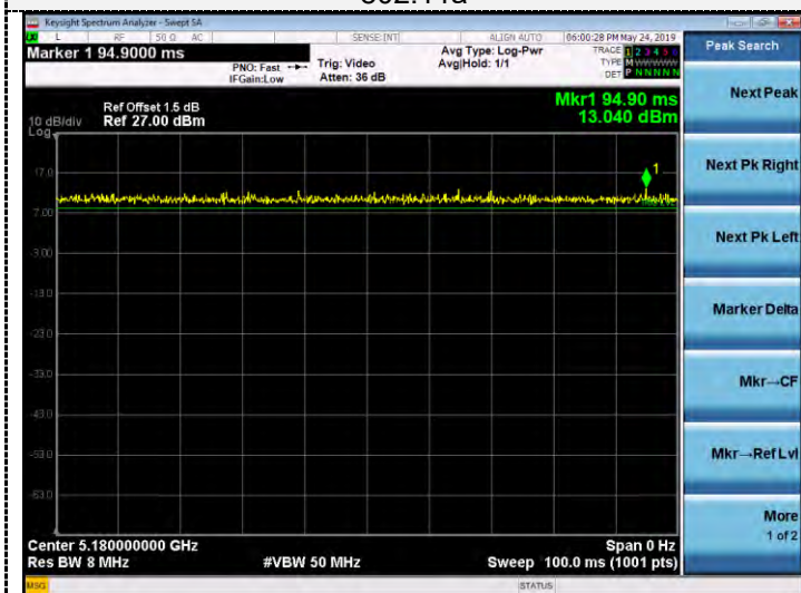
802.11a
