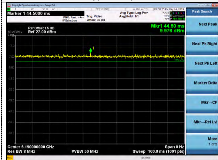
802.11ac40
