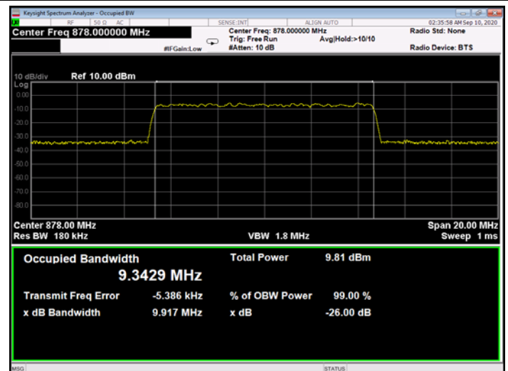
Figure 269: 256QAM 10MHz B.W.; 878.0MHz, 15kHz - Input
