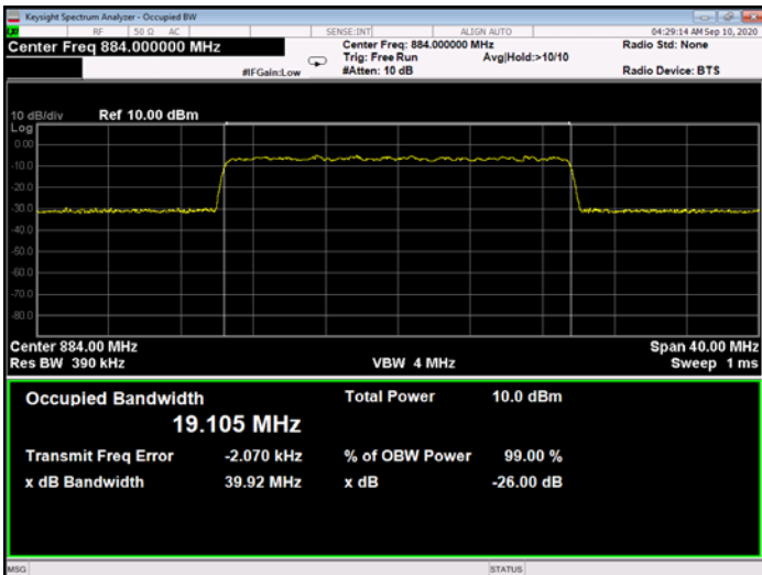
Figure 290: 256QAM 20MHz B.W.; 884.0MHz, 15kHz - Input
