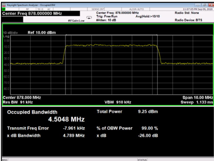
Figure 304: QPSK 5MHz B.W.; 878.0MHz, 15kHz - Input
