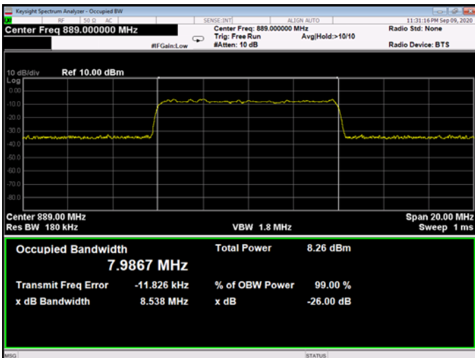
Figure 316: QPSK 10MHz B.W.; 889.0MHz, 60kHz - Input
