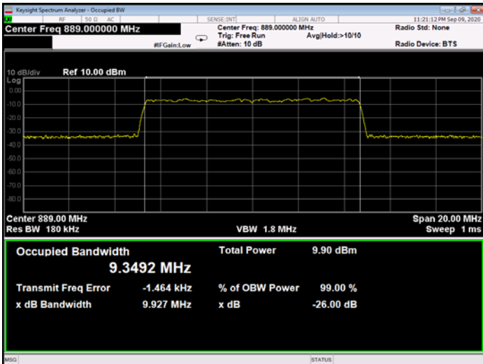
Figure 314: QPSK 10MHz B.W.; 889.0MHz, 15kHz - Input
