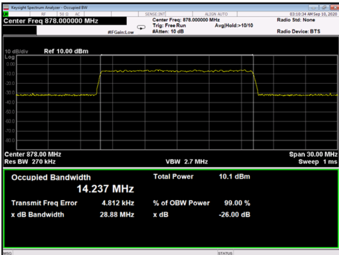
Figure 278: 256QAM 15MHz B.W.; 878.0MHz, 15kHz - Input
