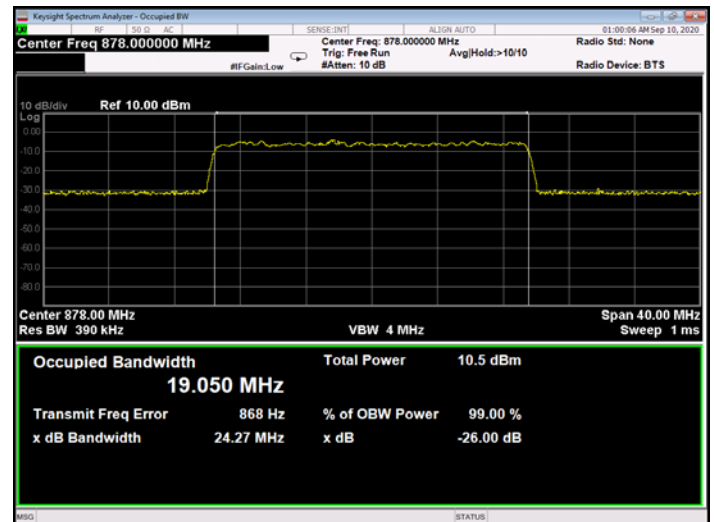
Figure 329: QPSK 20MHz B.W.; 878.0MHz, 15kHz - Input
