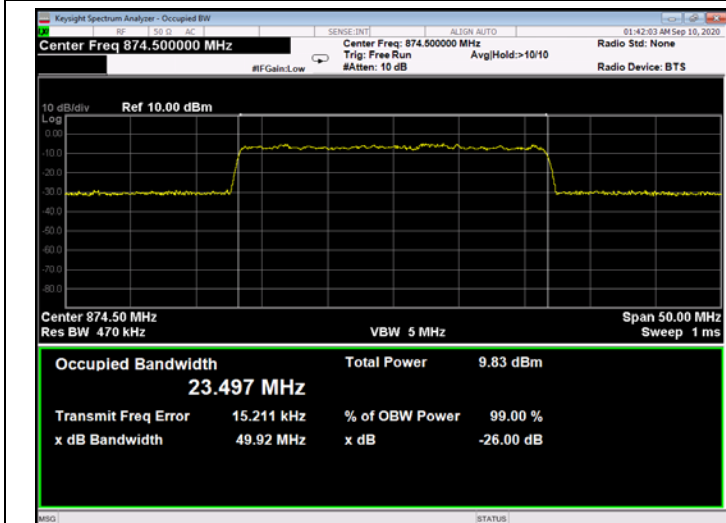
Figure 336: QPSK 25MHz B.W.; 874.5MHz, 30kHz - Input
