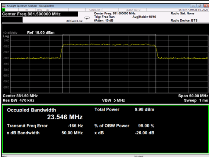
Figure 300: 256QAM 25MHz B.W.; 881.5MHz, 30kHz - Input
