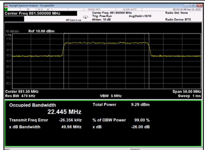
Figure 301: 256QAM 25MHz B.W.; 881.5MHz, 60kHz - Input
