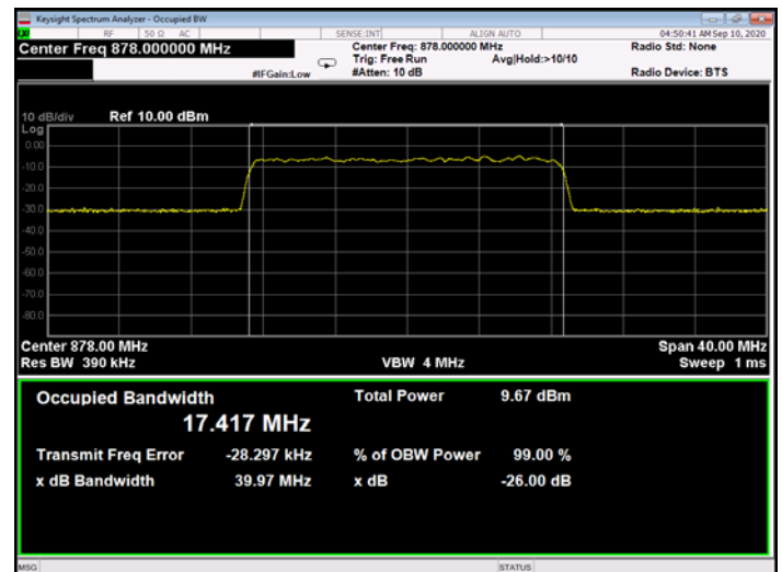
Figure 289: 256QAM 20MHz B.W.; 878.0MHz, 60kHz - Input
