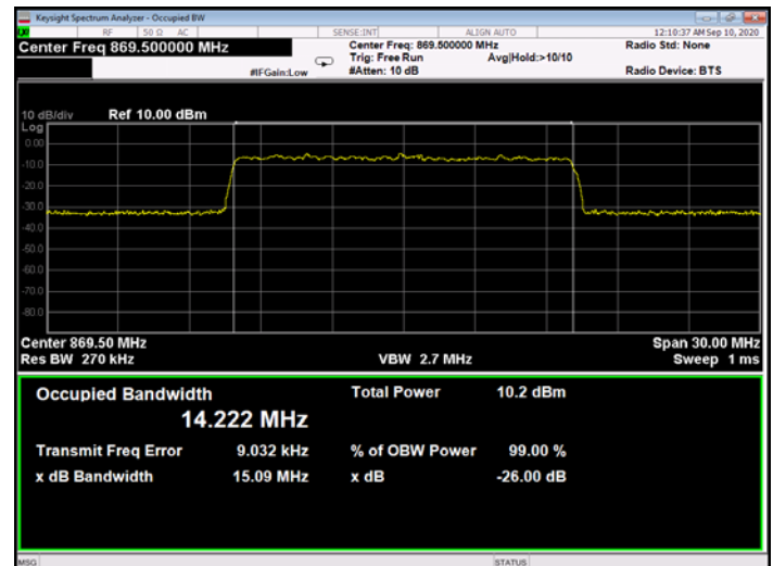
Figure 317: QPSK 15MHz B.W.; 869.5MHz, 15kHz - Input
