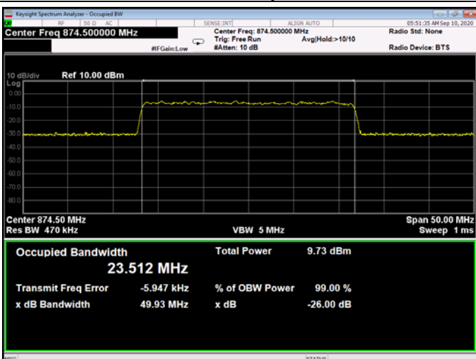
Figure 294: 256QAM 25MHz B.W.; 874.5MHz, 30kHz - Input
