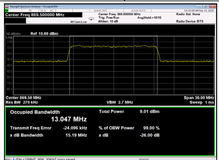
Figure 277: 256QAM 15MHz B.W.; 869.5MHz, 60kHz - Input
