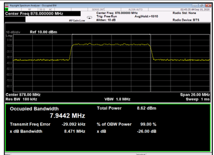
Figure 271: 256QAM 10MHz B.W.; 878.0MHz, 60kHz - Input
