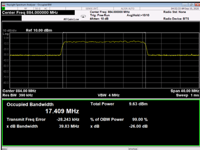
Figure 292: 256QAM 20MHz B.W.; 884.0MHz, 60kHz - Input
