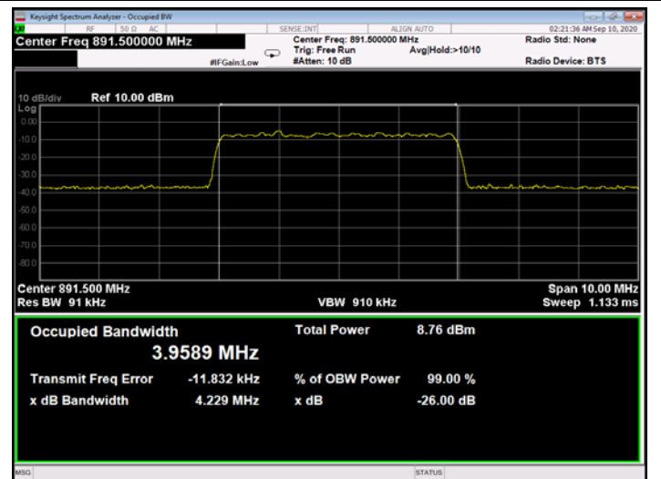
Figure 265: 256QAM 5MHz B.W.; 891.5MHz, 30kHz - Input
