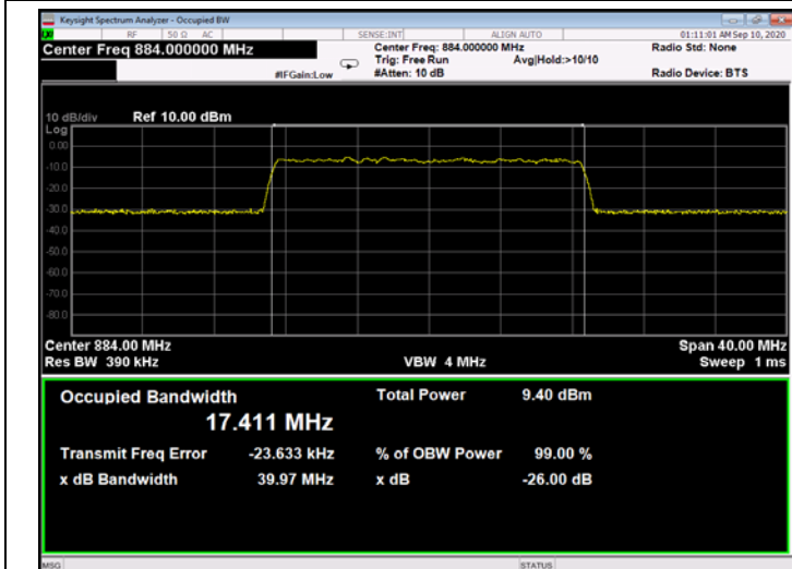
Figure 334: QPSK 20MHz B.W.; 884.0MHz, 60kHz - Input
