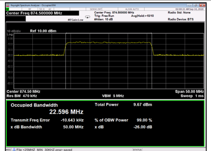
Figure 337: QPSK 25MHz B.W.; 874.5MHz, 60kHz - Input
