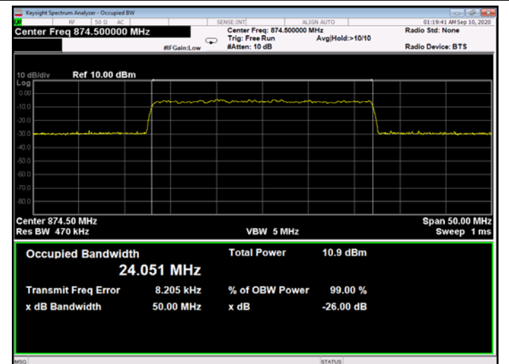
Figure 335: QPSK 25MHz B.W.; 874.5MHz, 15kHz - Input
