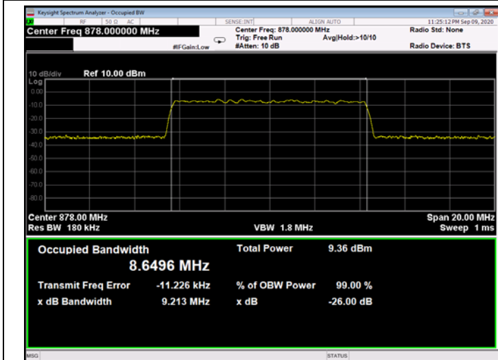
Figure 312: QPSK 10MHz B.W.; 878.0MHz, 30kHz - Input
