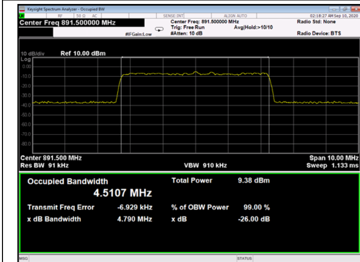
Figure 264: 256QAM 5MHz B.W.; 891.5MHz, 15kHz - Input
