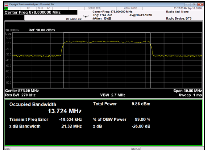
Figure 279: 256QAM 15MHz B.W.; 878.0MHz, 30kHz - Input
