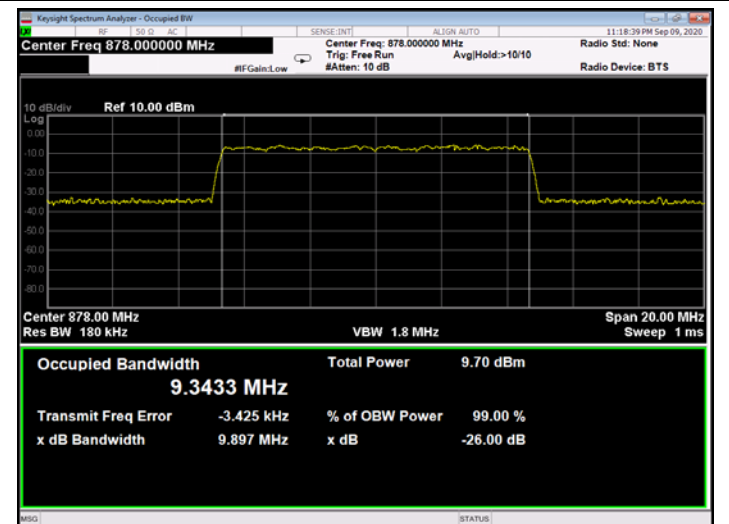
Figure 311: QPSK 10MHz B.W.; 878.0MHz, 15kHz - Input
