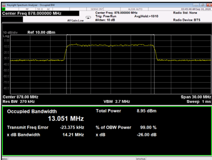
Figure 280: 256QAM 15MHz B.W.; 878.0MHz, 60kHz - Input
