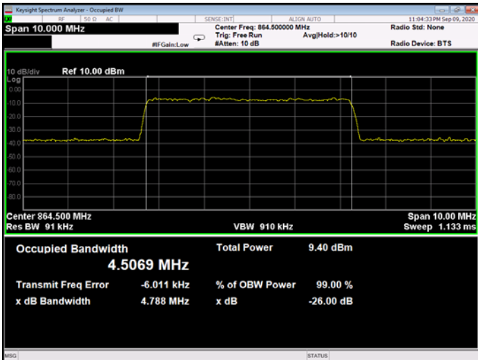
Figure 302: QPSK 5MHz B.W.; 864.5MHz, 15kHz - Input
