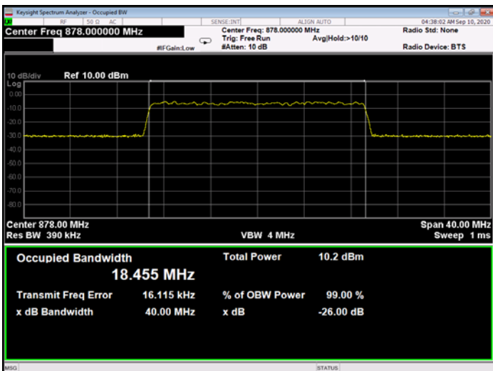
Figure 288: 256QAM 20MHz B.W.; 878.0MHz, 30kHz - Input
