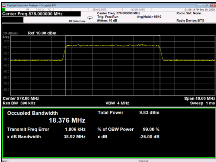
Figure 330: QPSK 20MHz B.W.; 878.0MHz, 30kHz - Input
