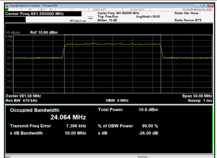
Figure 341: QPSK 25MHz B.W.; 881.5MHz, 15kHz - Input
