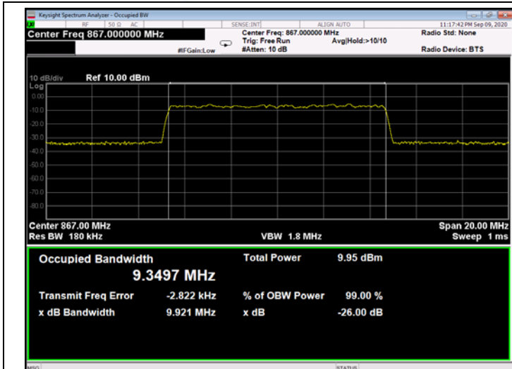
Figure 308: QPSK 10MHz B.W.; 867.0MHz, 15kHz - Input
