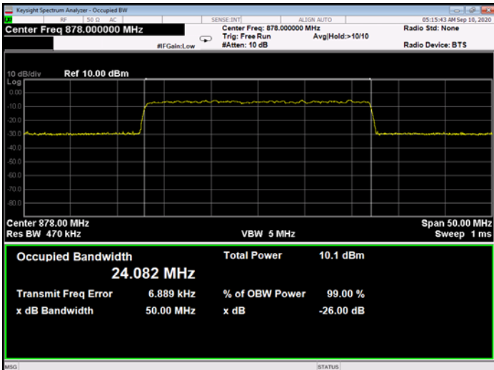
Figure 296: 256QAM 25MHz B.W.; 878.0MHz, 15kHz - Input
