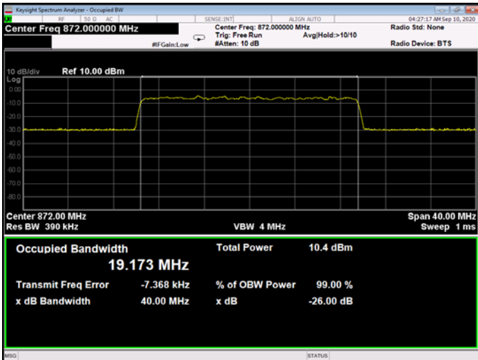
Figure 284: 256QAM 20MHz B.W.; 872.0MHz, 15kHz - Input
