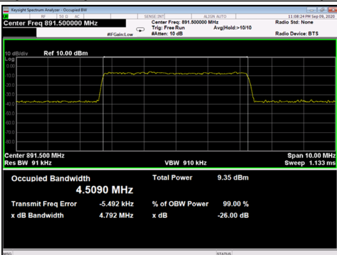
Figure 306: QPSK 5MHz B.W.; 891.50MHz, 15kHz - Input
