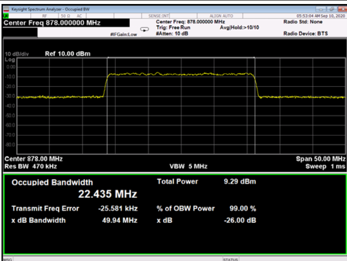
Figure 298: 256QAM 25MHz B.W.; 878.0MHz, 60kHz - Input
