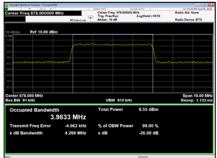
Figure 305: QPSK 5MHz B.W.; 878.0MHz, 30kHz - Input
