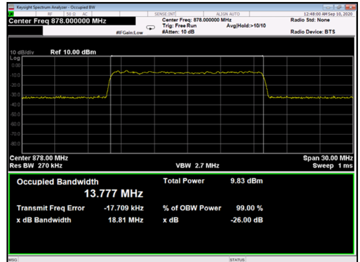
Figure 321: QPSK 15MHz B.W.; 878.0MHz, 30kHz - Input
