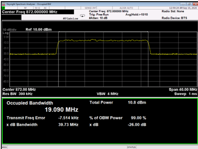
Figure 326: QPSK 20MHz B.W.; 872.0MHz, 15kHz - Input
