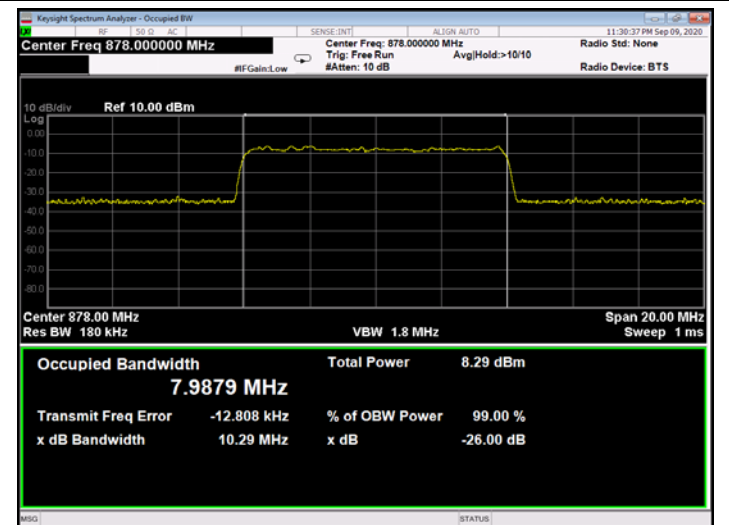
Figure 313: QPSK 10MHz B.W.; 878.0MHz, 60kHz - Input
