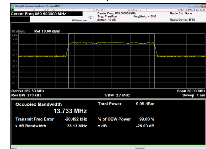
Figure 276: 256QAM 15MHz B.W.; 869.5MHz, 30kHz - Input
