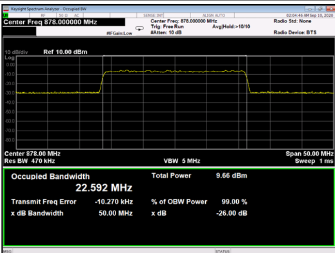
Figure 340: QPSK 25MHz B.W.; 878.0MHz, 60kHz - Input
