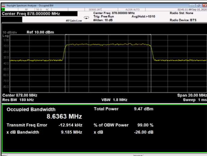
Figure 270: 256QAM 10MHz B.W.; 878.0MHz, 30kHz - Input
