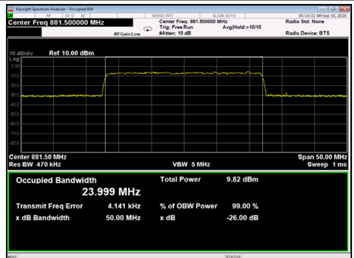
Figure 299: 256QAM 25MHz B.W.; 881.5MHz, 15kHz - Input
