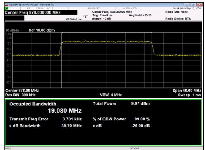
Figure 287: 256QAM 20MHz B.W.; 878.0MHz, 15kHz - Input
