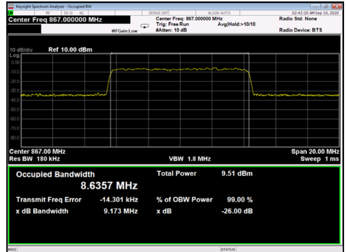
Figure 267: 256QAM 10MHz B.W.; 867.0MHz, 30kHz - Input
