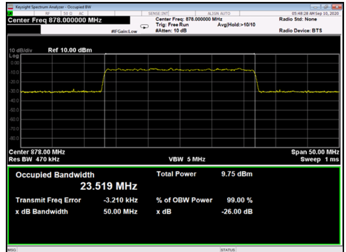
Figure 297: 256QAM 25MHz B.W.; 878.0MHz, 30kHz - Input
