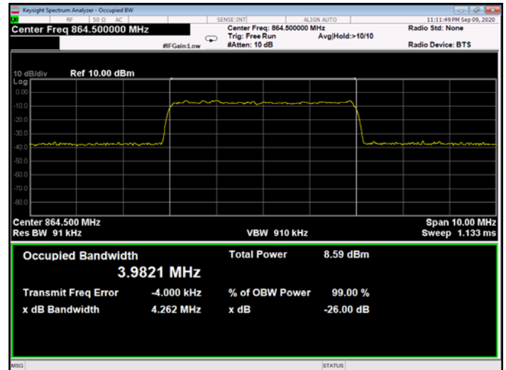
Figure 303: QPSK 5MHz B.W.; 864.5MHz, 30kHz - Input
