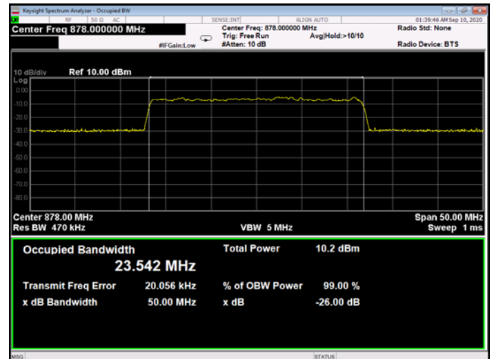
Figure 339: QPSK 25MHz B.W.; 878.0MHz, 30kHz - Input
