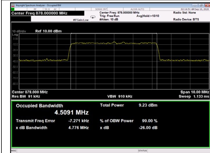
Figure 262: 256QAM 5MHz B.W.; 878.0MHz, 15kHz - Input
