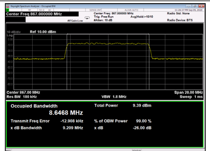
Figure 309: QPSK 10MHz B.W.; 867.0MHz, 30kHz - Input
