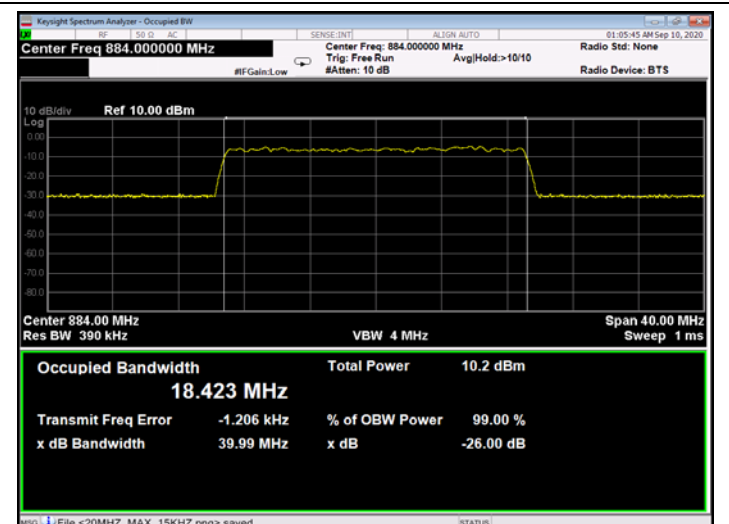
Figure 333: QPSK 20MHz B.W.; 884.0MHz, 30kHz - Input
