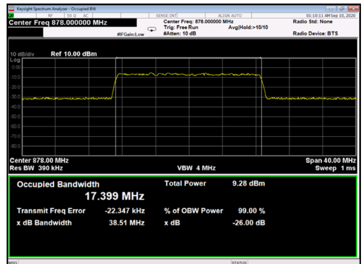
Figure 331: QPSK 20MHz B.W.; 878.0MHz, 60kHz - Input
