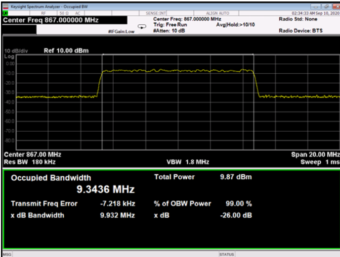
Figure 266: 256QAM 10MHz B.W.; 867.0MHz, 15kHz - Input
