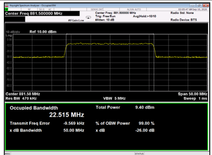
Figure 343: QPSK 25MHz B.W.; 881.5MHz, 60kHz - Input
