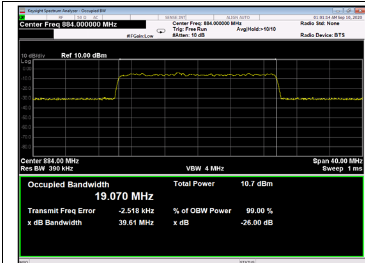
Figure 332: QPSK 20MHz B.W.; 884.0MHz, 15kHz - Input
