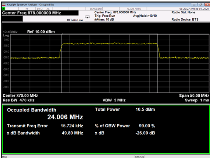
Figure 338: QPSK 25MHz B.W.; 878.0MHz, 15kHz - Input
