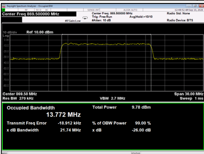
Figure 318: QPSK 15MHz B.W.; 869.5MHz, 30kHz - Input
