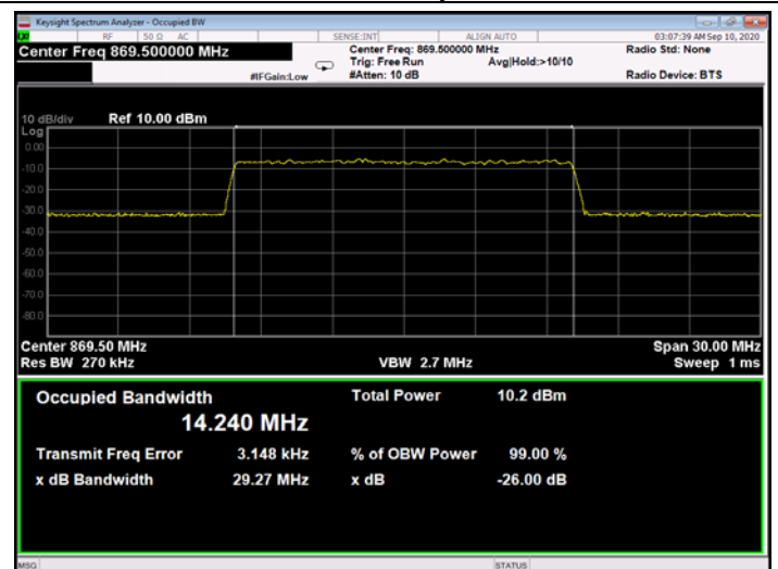
Figure 275: 256QAM 15MHz B.W.; 869.5MHz, 15kHz - Input
