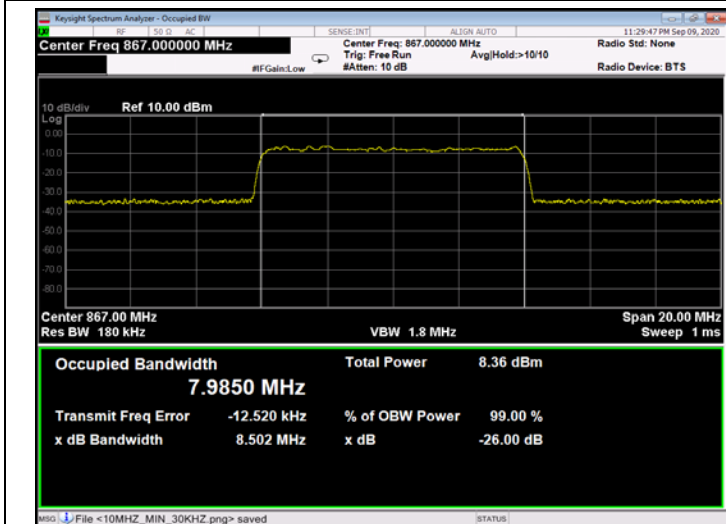
Figure 310: QPSK 10MHz B.W.; 867.0MHz, 60kHz - Input
