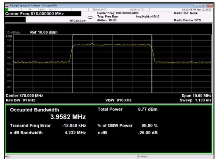
Figure 263: 256QAM 5MHz B.W.; 878.0MHz, 30kHz - Input
