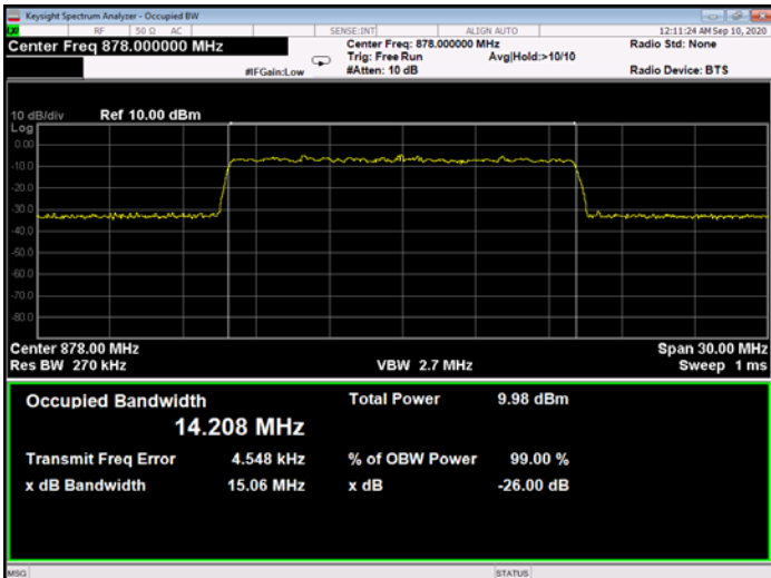
Figure 320: QPSK 15MHz B.W.; 878.0MHz, 15kHz - Input
