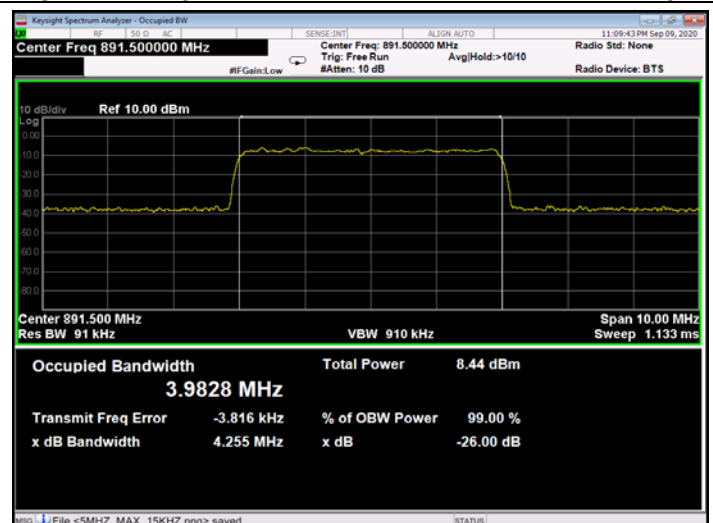
Figure 307: QPSK 5MHz B.W.; 891.5MHz, 30kHz - Input
