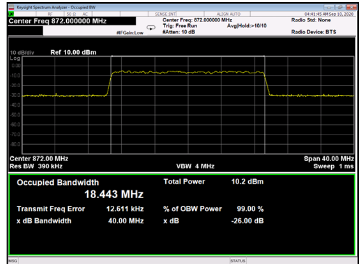
Figure 285: 256QAM 20MHz B.W.; 872.0MHz, 30kHz - Input
