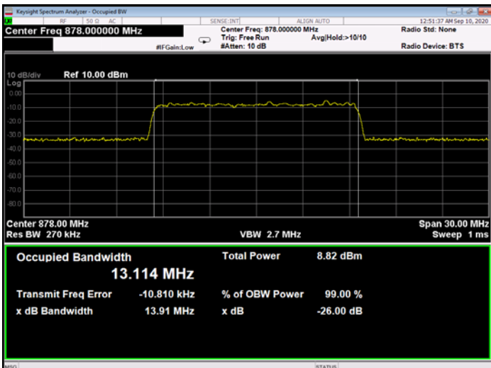
Figure 322: QPSK 15MHz B.W.; 878.0MHz, 60kHz - Input
