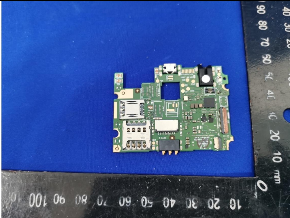
MT6739
