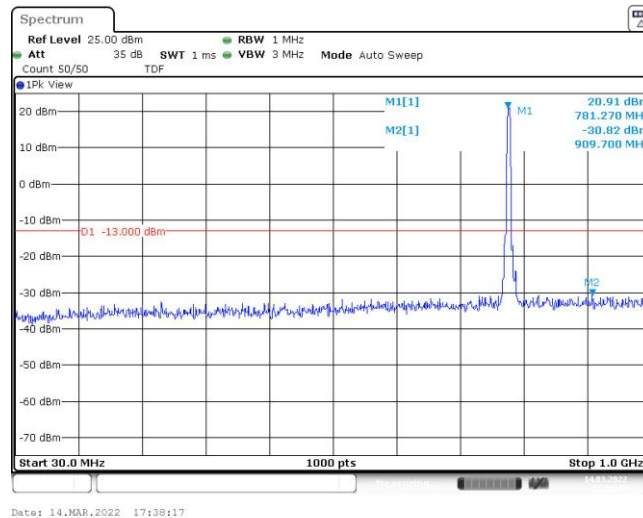
Band13-5MHz-QPSK-23230-25RB#0-Range1:30~1000MHz
