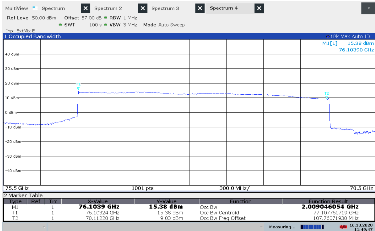
Plot 54: OBW, +40 °C / V nom , Mode 6
