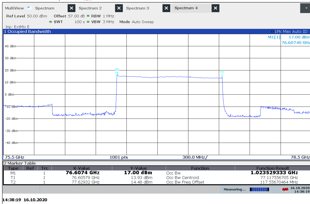
Plot 15: Mode 3 – OBW, T_{\min} / V_{\text{nom}}
