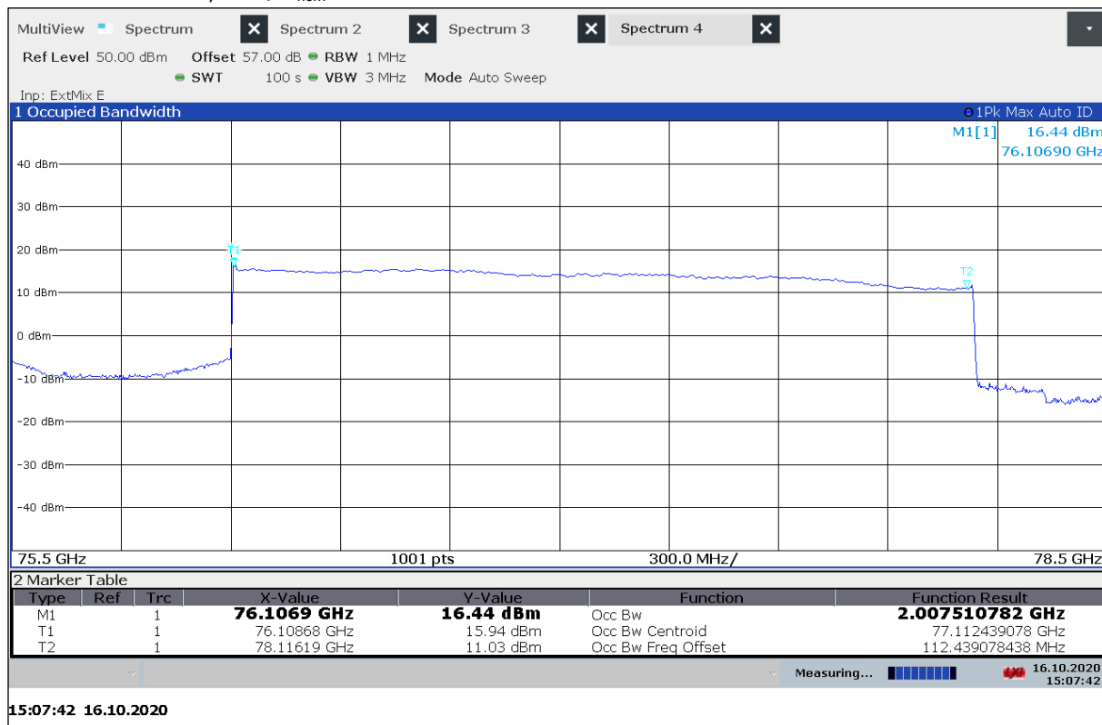
Plot 16: Mode 6 – OBW, T_{\min} / V_{\text{nom}}
