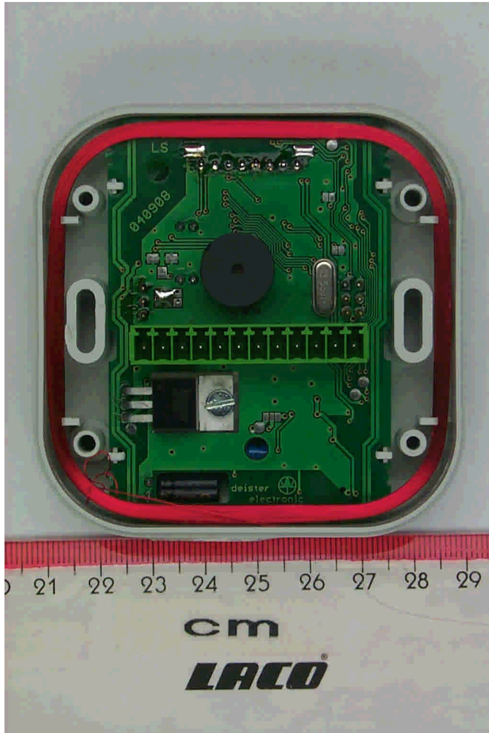
41092C_f.jpg KPD5 / SWH-4200, rear view
