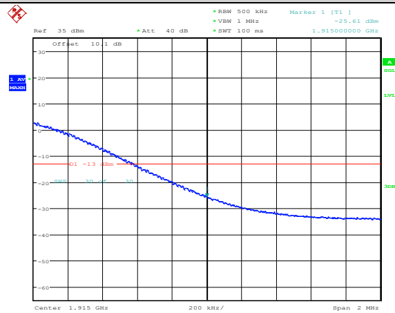
Band25-20MHz-QPSK-26590-100RB#0
