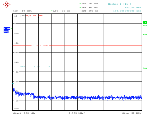
Band25-1.4MHz-QPSK-26047-1RB#0-Range2:0.15~30MHz
