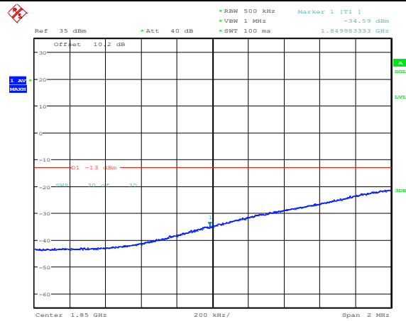
Band25-20MHz-QPSK-26140-1RB#99
