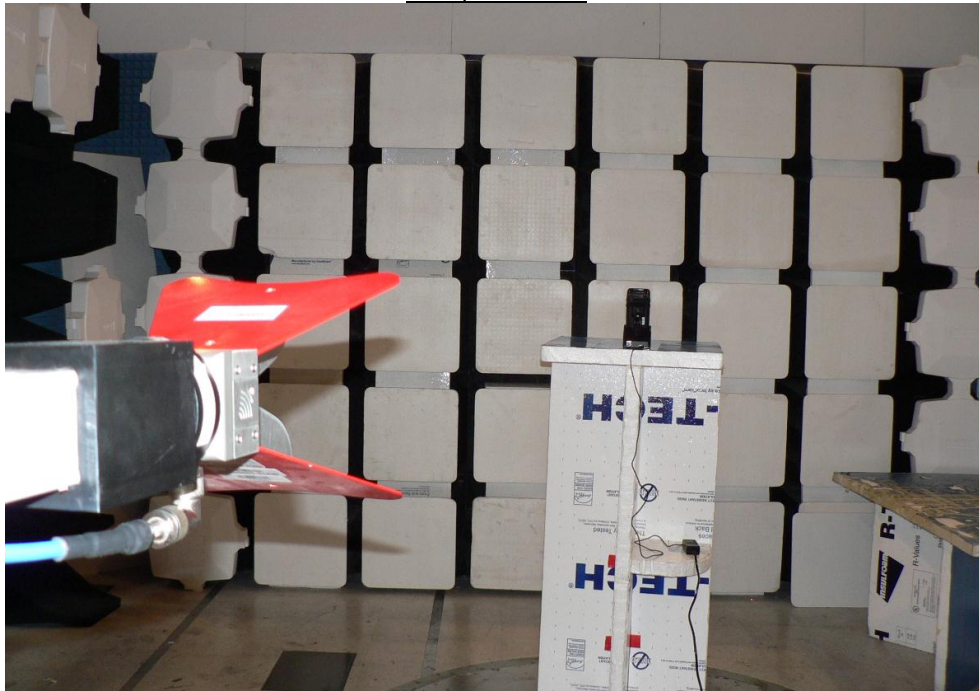
TX Spur 1-18G
