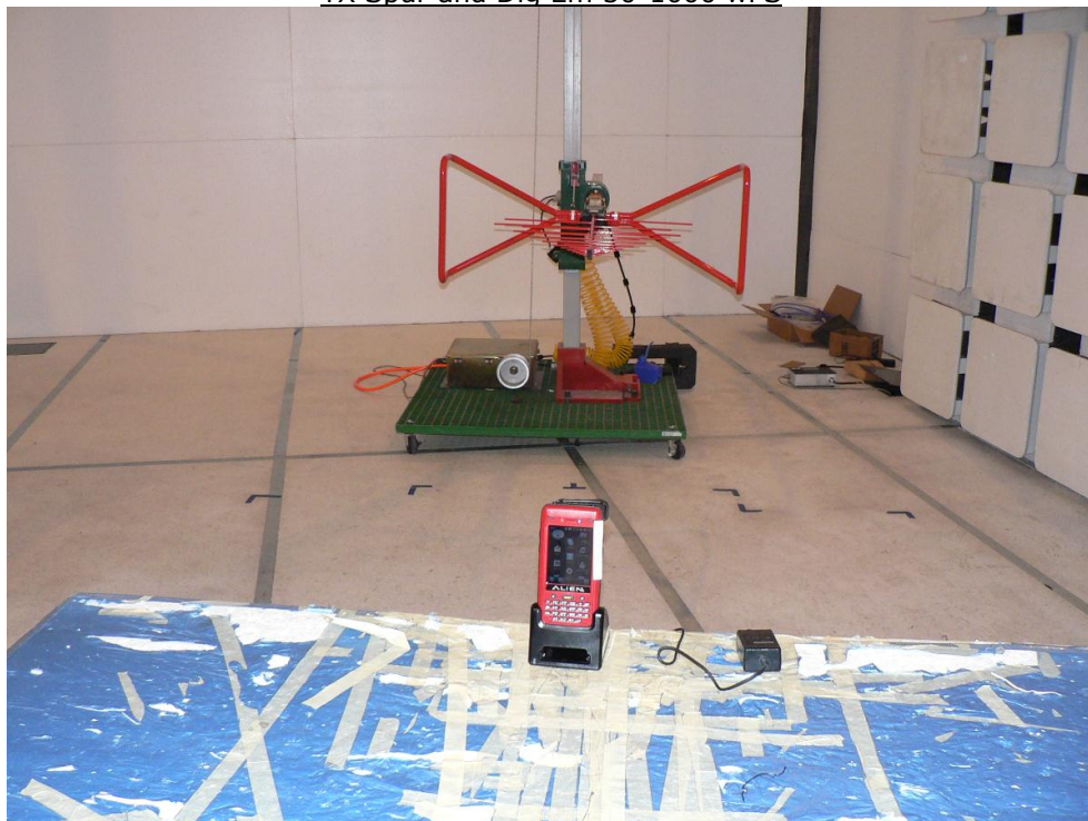
TX Spur and Dig Em 30-1000 wPS
