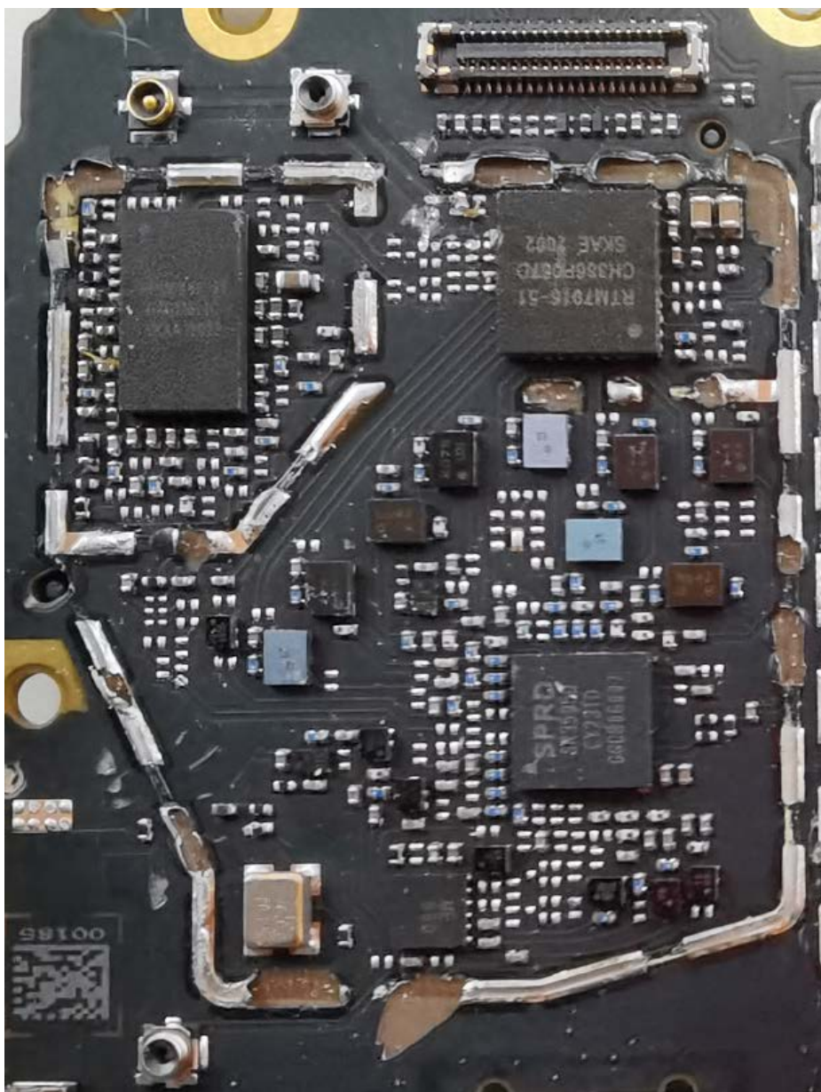
IC Details 9
