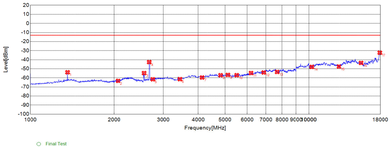
CH 128400 20M CP-OFDM QPSK 1RB_Left SCS 15KHz 1-18G V
