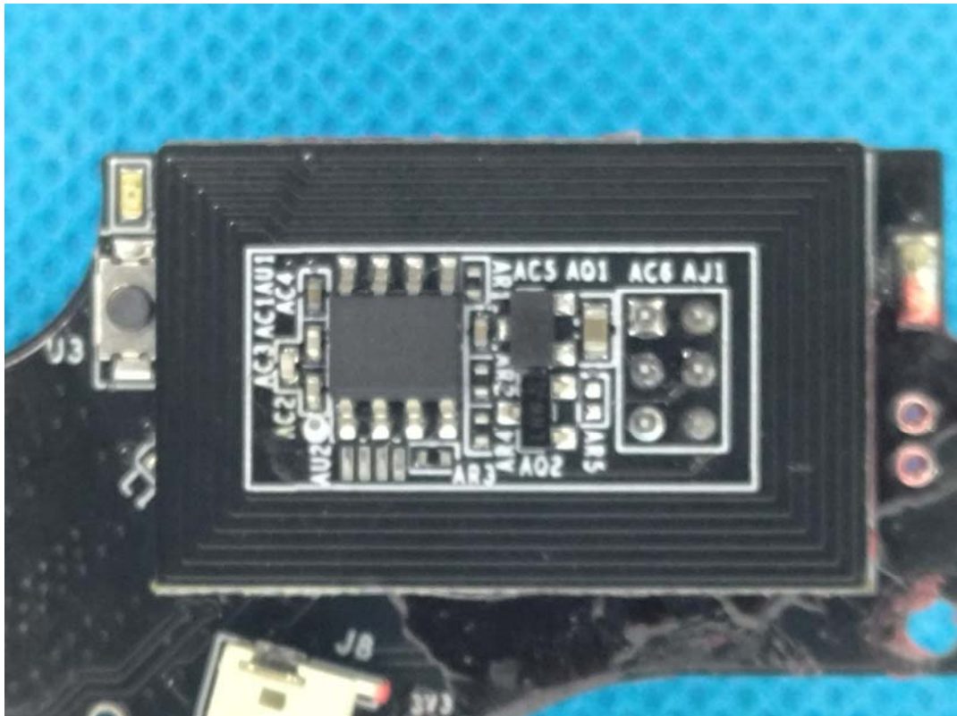
NFC Antenna
