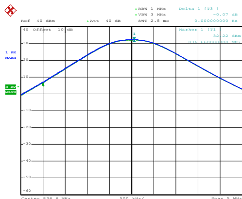
GSM 850
