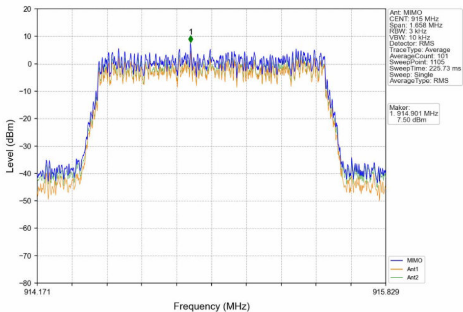
QPSK_MCH_915MHz_MIMO_NTNV
