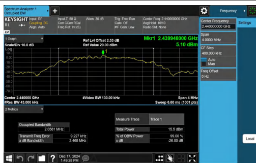
BLE_2M-Ant1-2440
