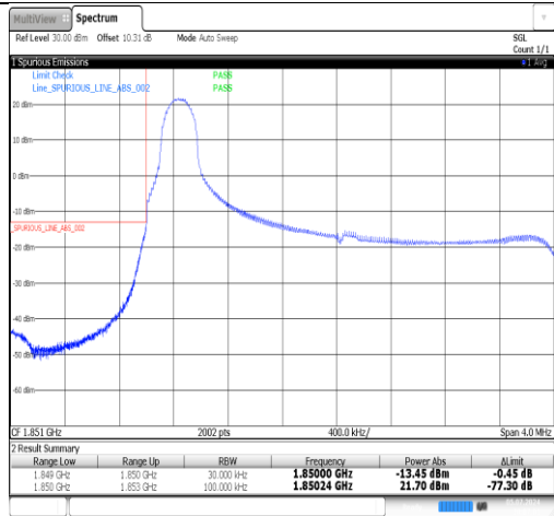
Band2-3MHz-16QAM-18615-1RB#14-PASS
