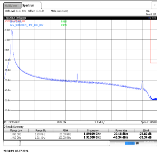
Band2-20MHz-16QAM-19100-1RB#99-PASS
