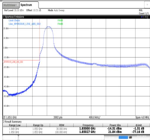
Band2-3MHz-QPSK-18615-1RB#14-PASS
