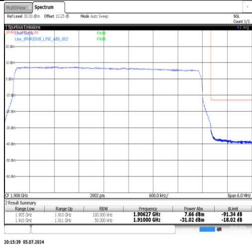
Band2-5MHz-16QAM-18625-1RB#0-PASS
