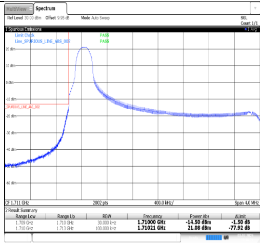
Band4-3MHz-QPSK-19965-1RB#14-PASS
