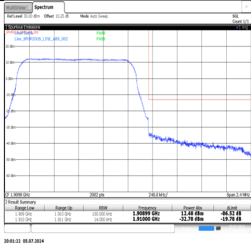
Band2-3MHz-QPSK-18615-1RB#0-PASS
