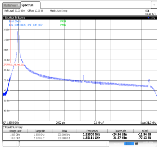
Band2-20MHz-QPSK-18700-1RB#99-PASS
