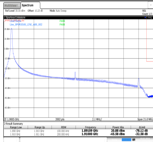
Band2-20MHz-QPSK-19100-1RB#99-PASS
