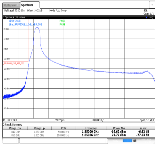
Band2-5MHz-QPSK-18625-1RB#24-PASS
