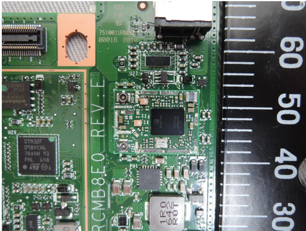
WLAN / BT Module - 2 (Model No.: QCNFA324)
