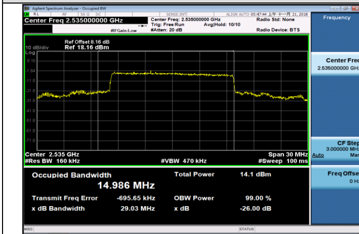
MCH_QPSK_75RB#0
