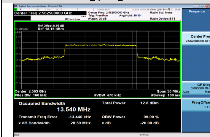
HCH_QPSK_75RB#0
