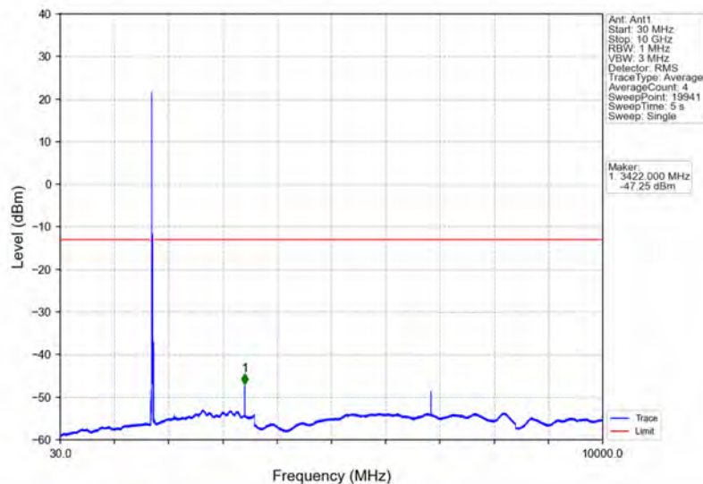
Band66_20MHz_16QAM_LCH_1720MHz_RB_1_0_NTNV
