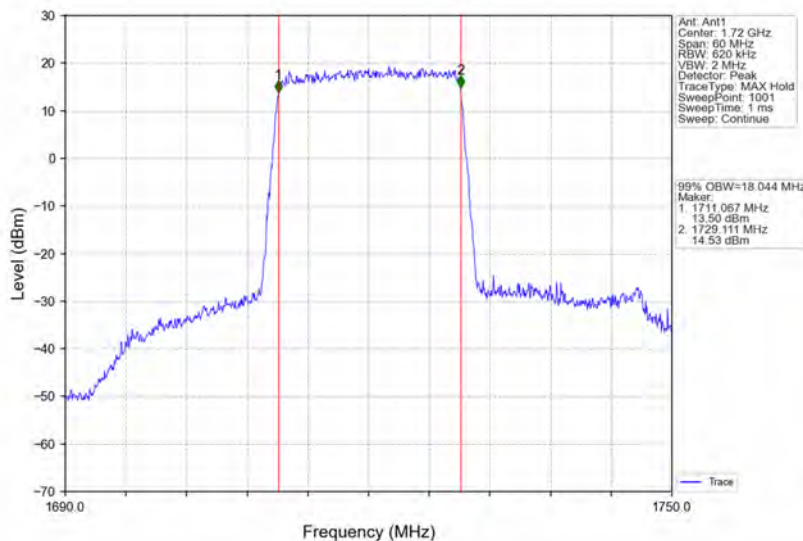
Band66_20MHz_QPSK_LCH_1720MHz_RB_100_0_NTNV
