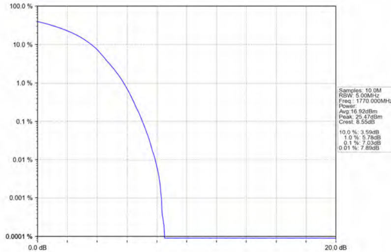
Band66_20MHz_QPSK_HCH_1770MHz_RB_100_0_NTNV
