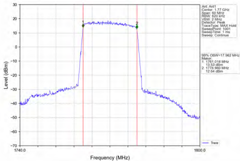
Band66_20MHz_QPSK_HCH_1770MHz_RB_100_0_NTNV
