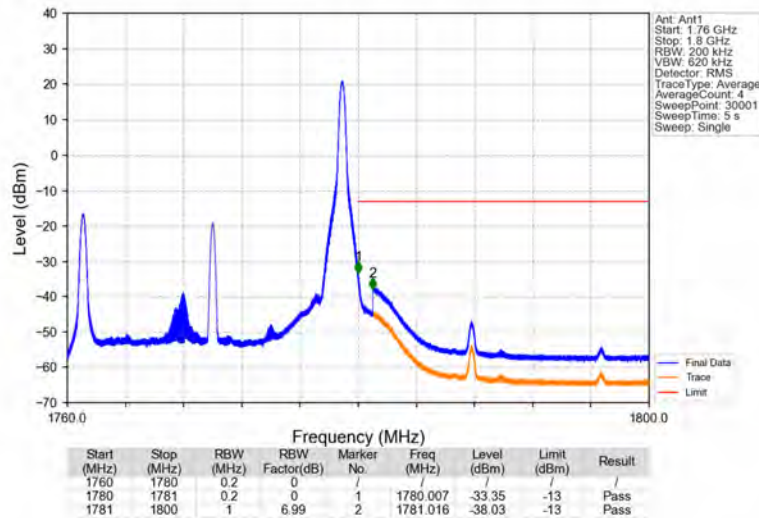
Band66_20MHz_QPSK_HCH_1770MHz_RB_1_99_NTNV
