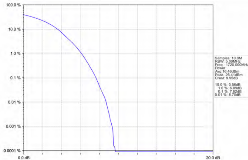
Band66_20MHz_16QAM_LCH_1720MHz_RB_100_0_NTNV
