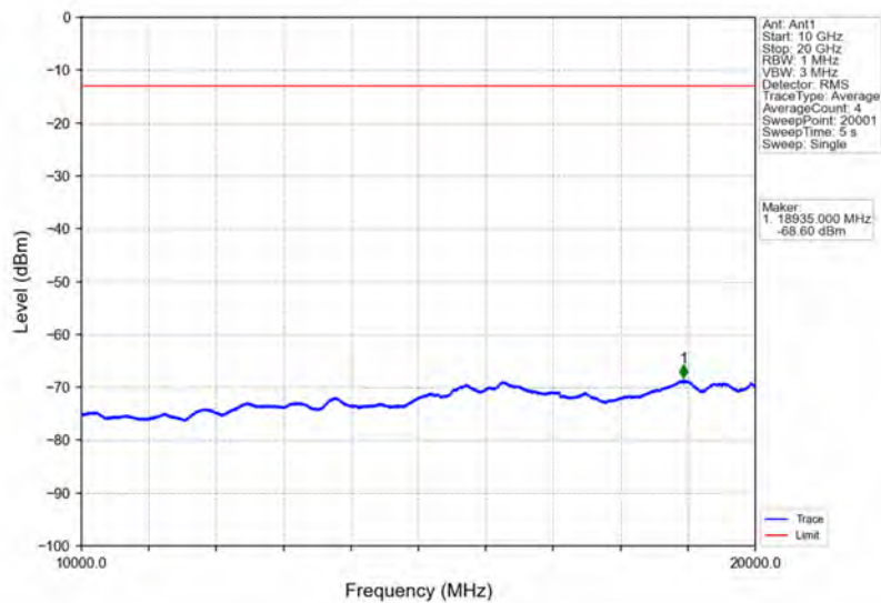
Band66_20MHz_QPSK_HCH_1770MHz_RB_1_0_NTNV
