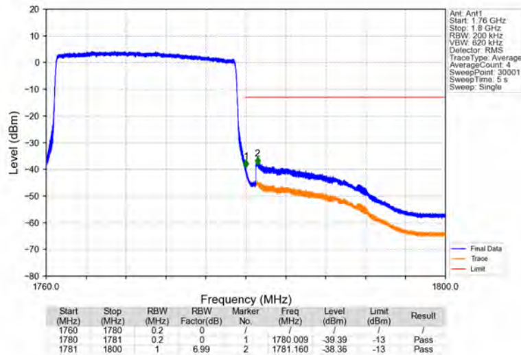
Band66_20MHz_QPSK_HCH_1770MHz_RB_100_0_NTNV
