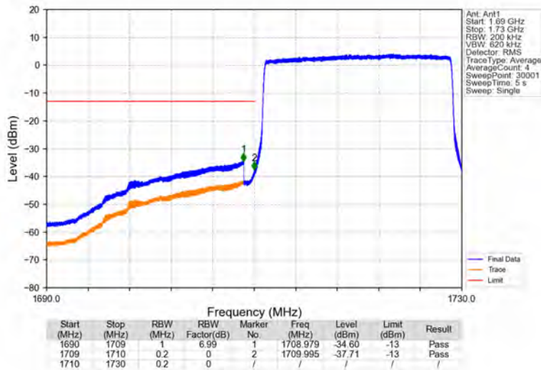
Band66_20MHz_16QAM_LCH_1720MHz_RB_100_0_NTNV
