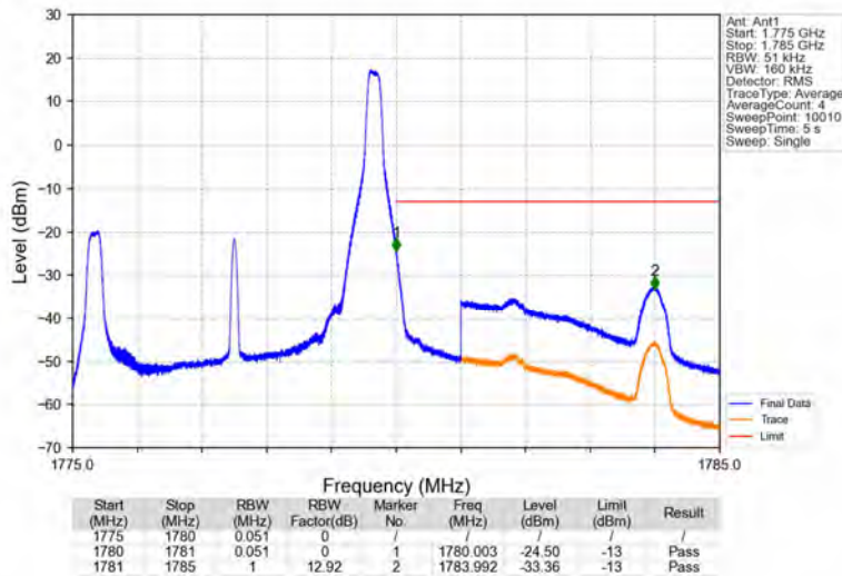
Band66_5MHz_QPSK_HCH_1777.5MHz_RB_1_24_NTNV
