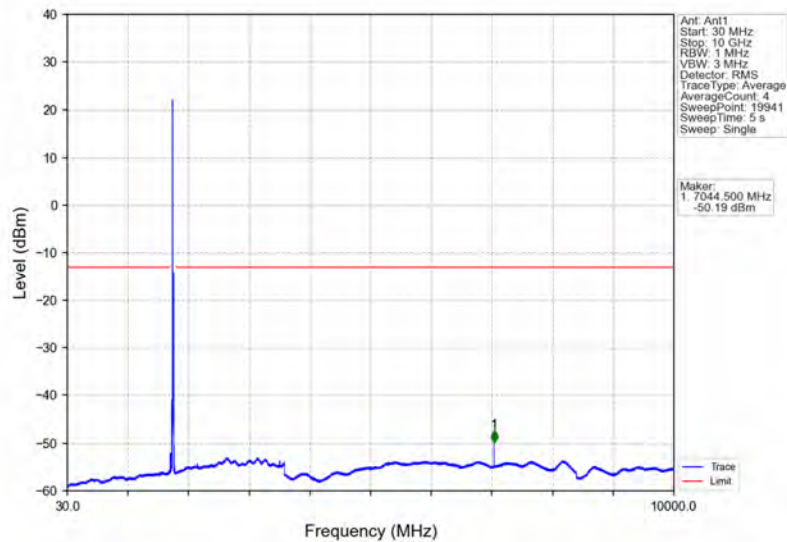
Band66_20MHz_QPSK_HCH_1770MHz_RB_1_0_NTNV
