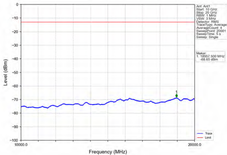
Band66_20MHz_QPSK_MCH_1745MHz_RB_1_0_NTNV
