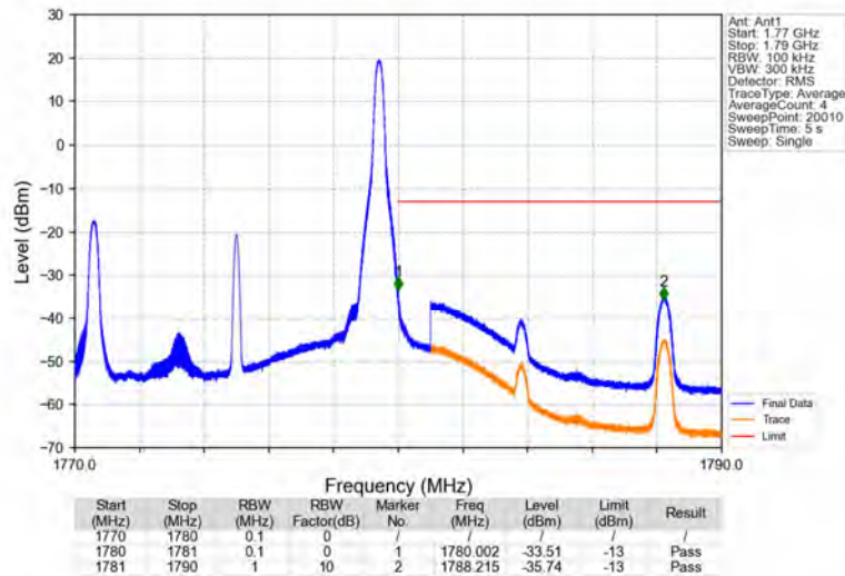
Band66_10MHz_QPSK_HCH_1775MHz_RB_1_49_NTNV
