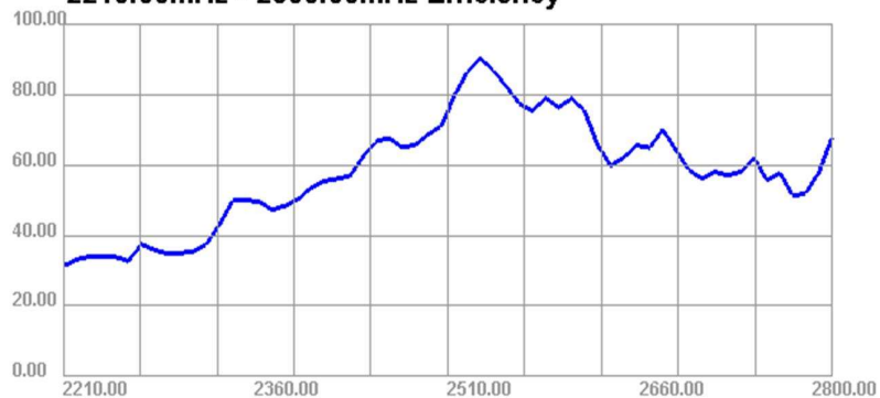
2210.00MHz - 2800.00MHz Efficiency
