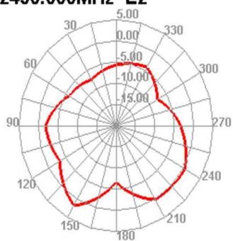
2450.000MHz E2
