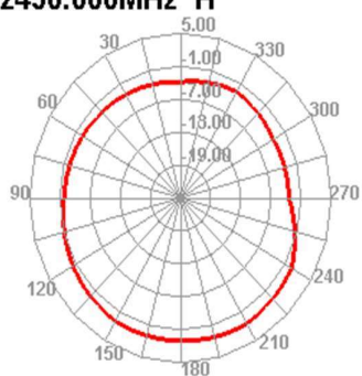
2450.000MHz H
