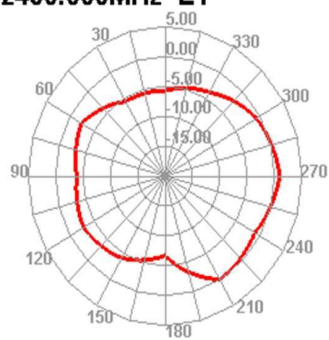
2450.000MHz E1
